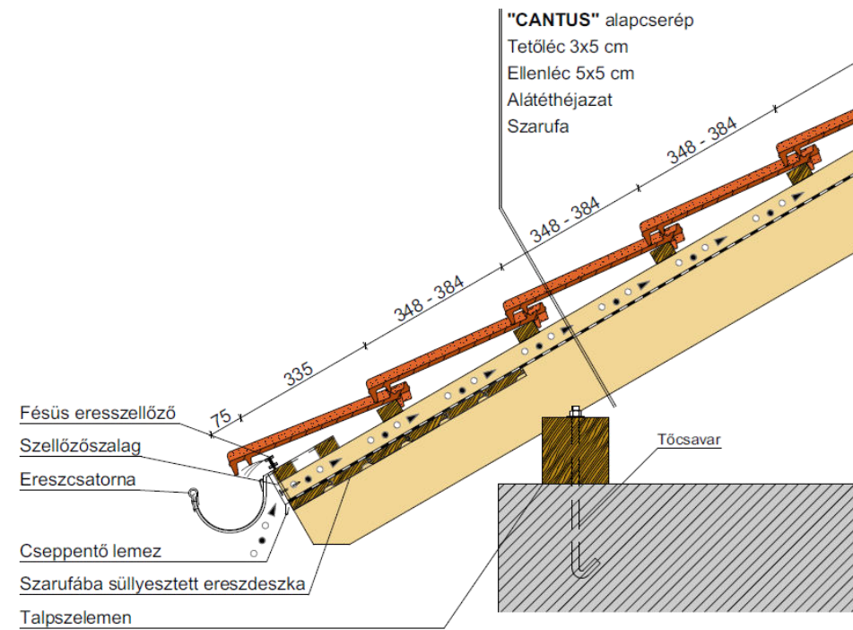
Ereszkialakítás
