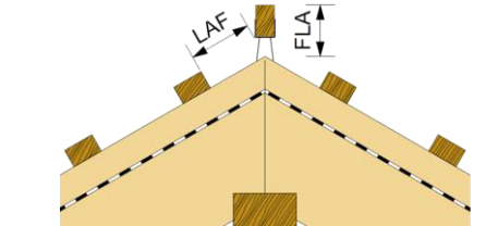
LAF: felső léc távolsága a gerinccsúctól FLA: gerincléc magassága a gerinccsúctól
