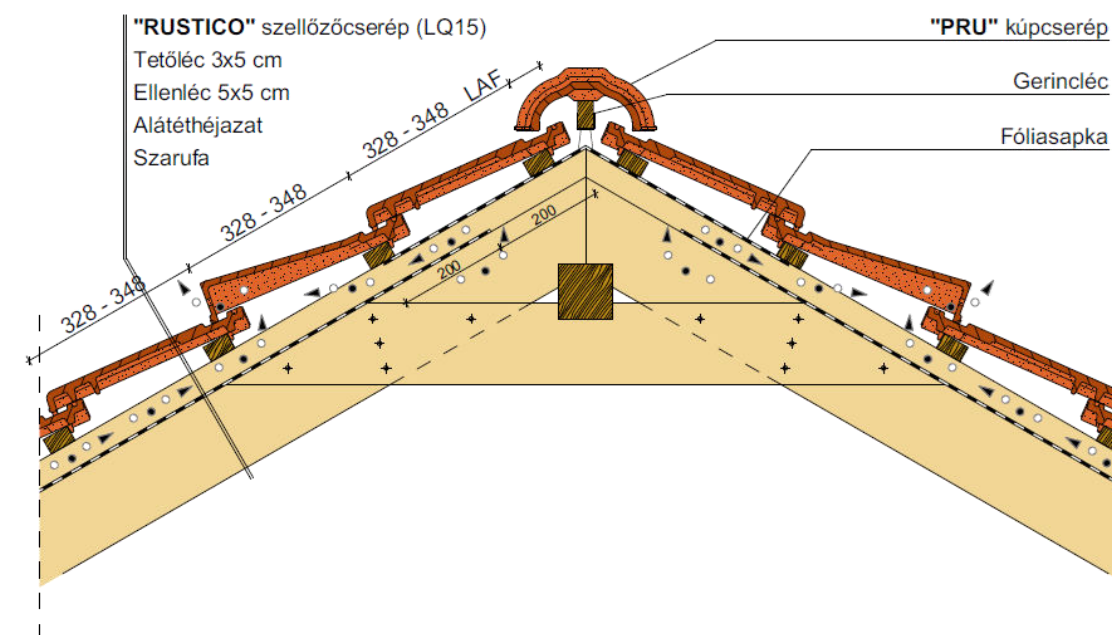
Gerinckialakítás, szellőzőcseréppel
