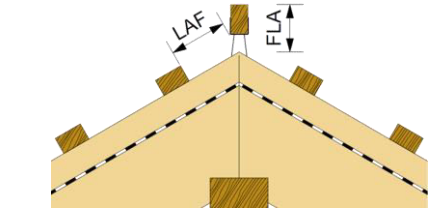
LAF: felső lécz távolsága a gerinccsúctól FLA: gerincléc magassága a gerinccsúctól
