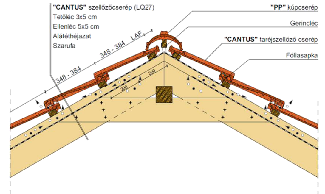
Gerinckialakítás, szellőzőcseréppel
