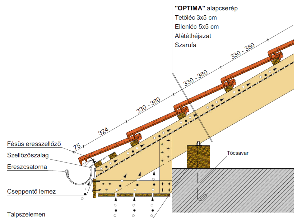
Dobozolt ereszkialakítás
