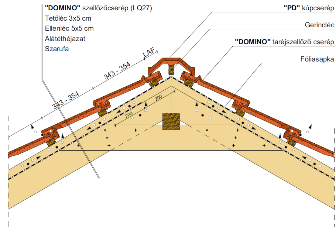
Gerinckialakítás, szellőzőcseréppel
