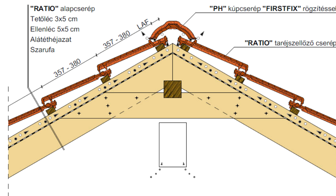
Gerinckialakítás, taréjszellőző cseréppel
