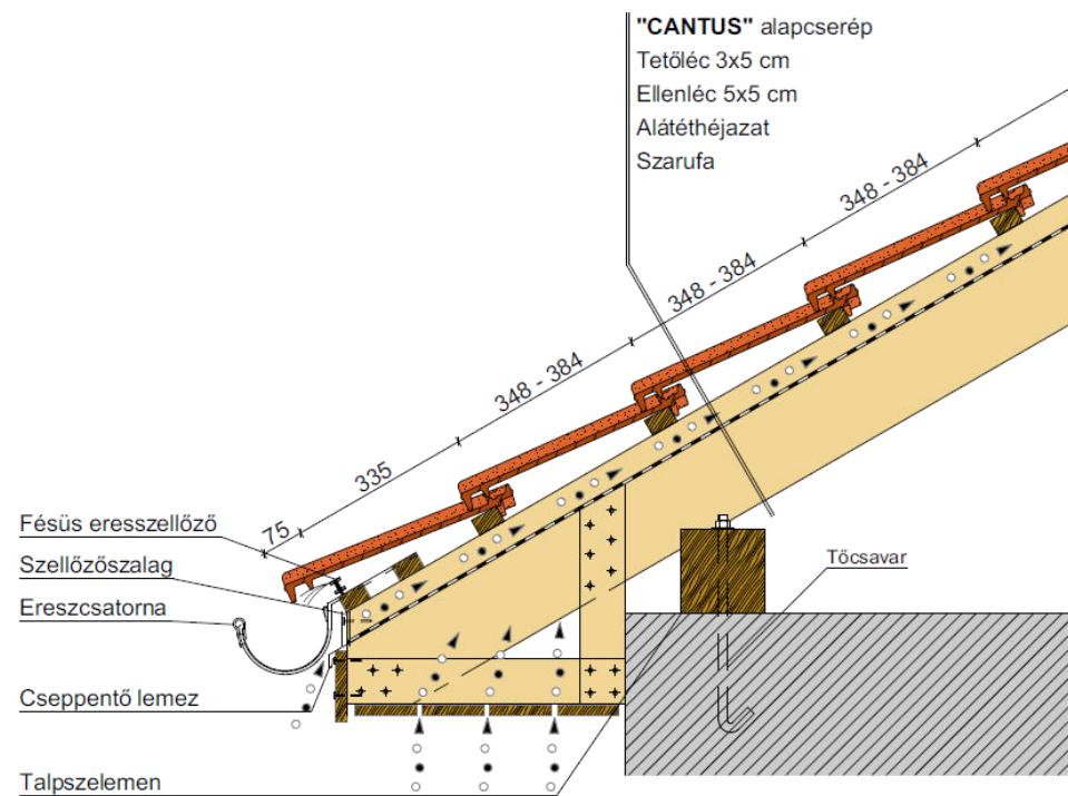
Dobozolt ereszkialakítás
