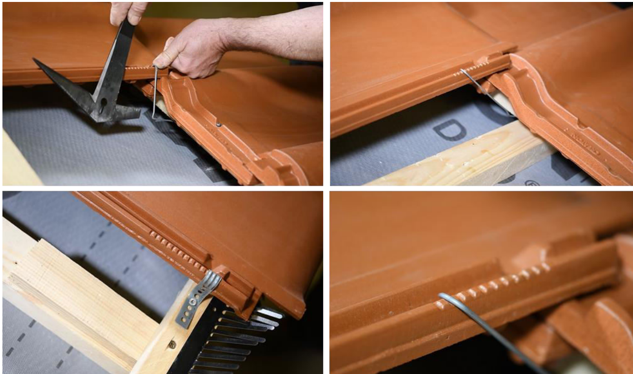
Beütős, beakasztós és az univerzális viharkapocs beépítése, továbbá beakasztós viharkapcsoknak kialakított barázdasor az oldalhoronyban
