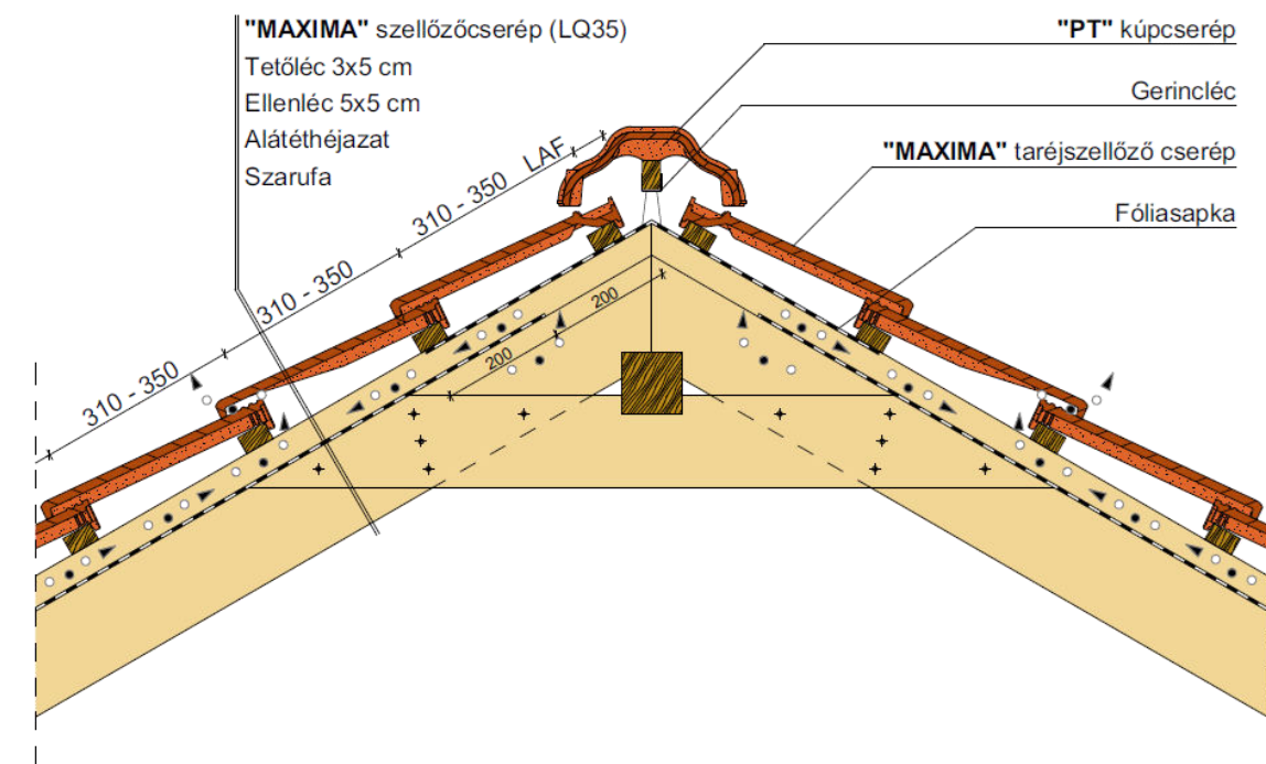
Gerinckialakítás, szellőzőcseréppel
