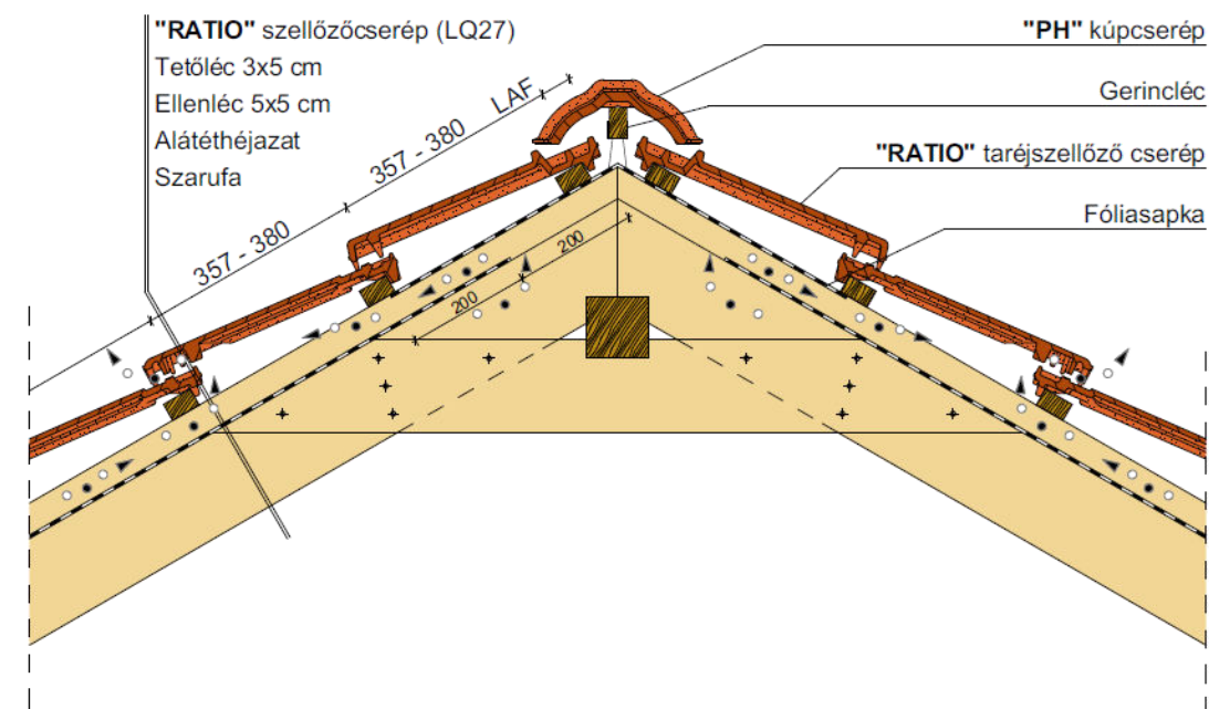
Gerinckialakítás, szellőzőcseréppel
