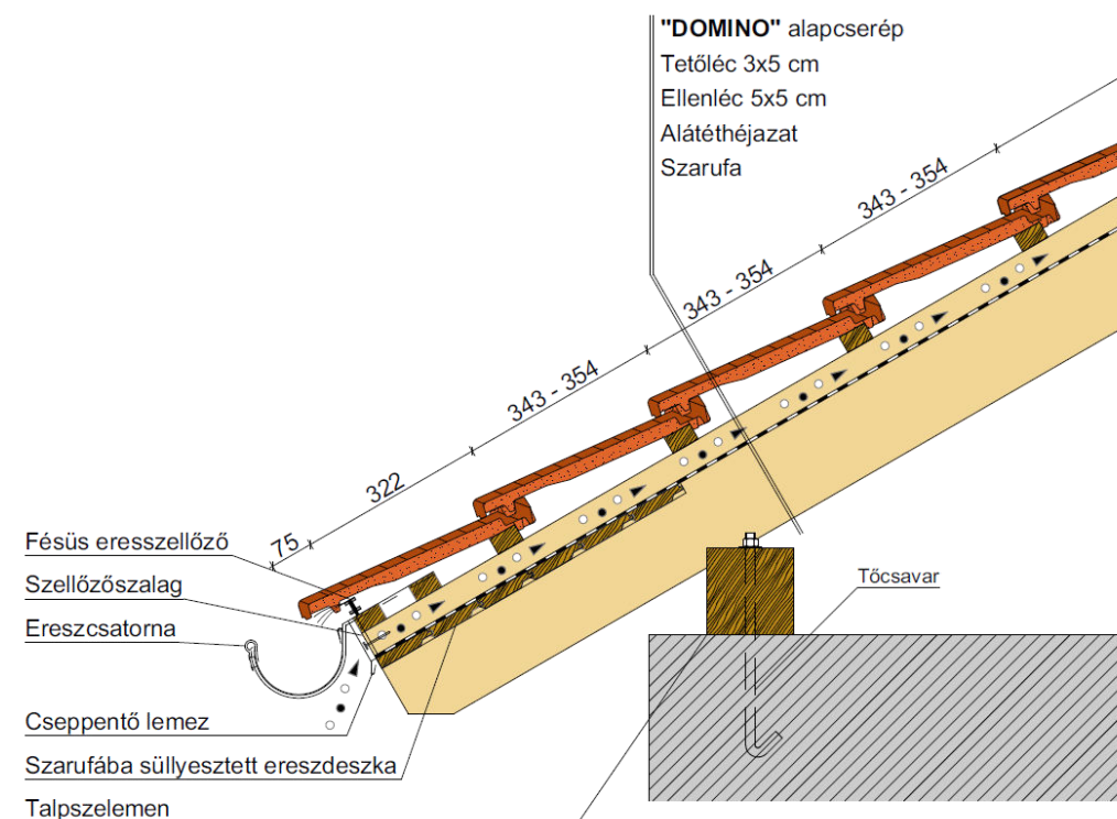
Ereszkialakítás
