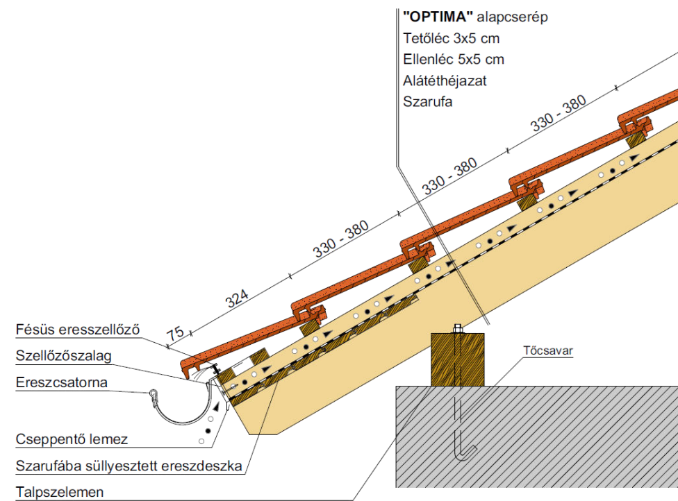
Ereszkialakítás
