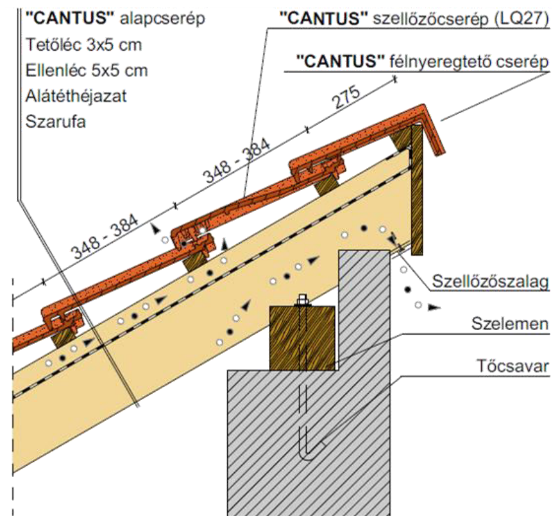
Félnyeregterítő gerinc, félnyeregterítő cseréppel
