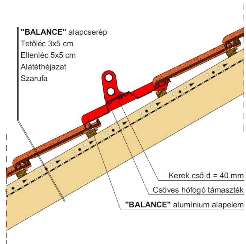
Hófogócső elhelyezése
