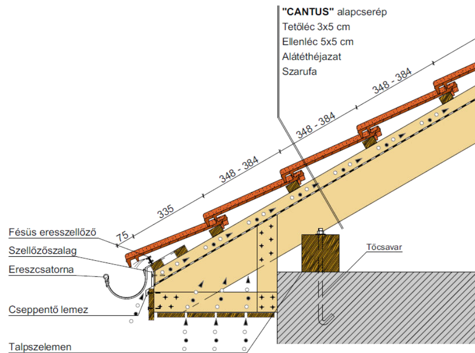
Dobozolt ereszkialakítás
