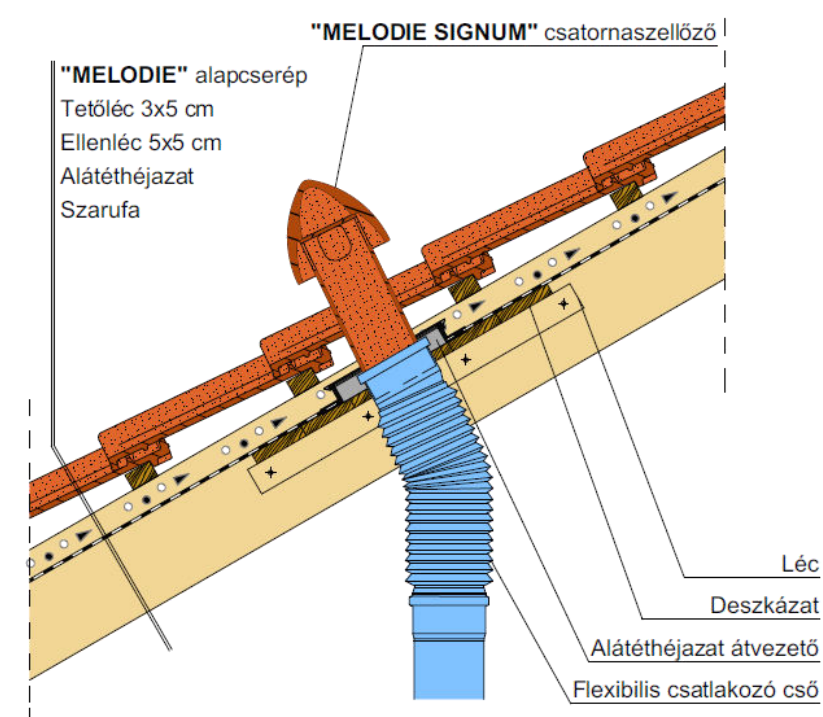
Kerámia csatornaszellőző átvezetés
