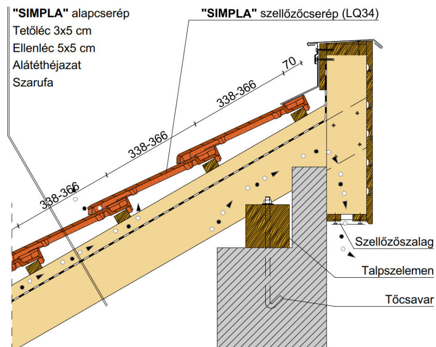
Félnyeregvető gerinc, félnyeregvető cseréppel
