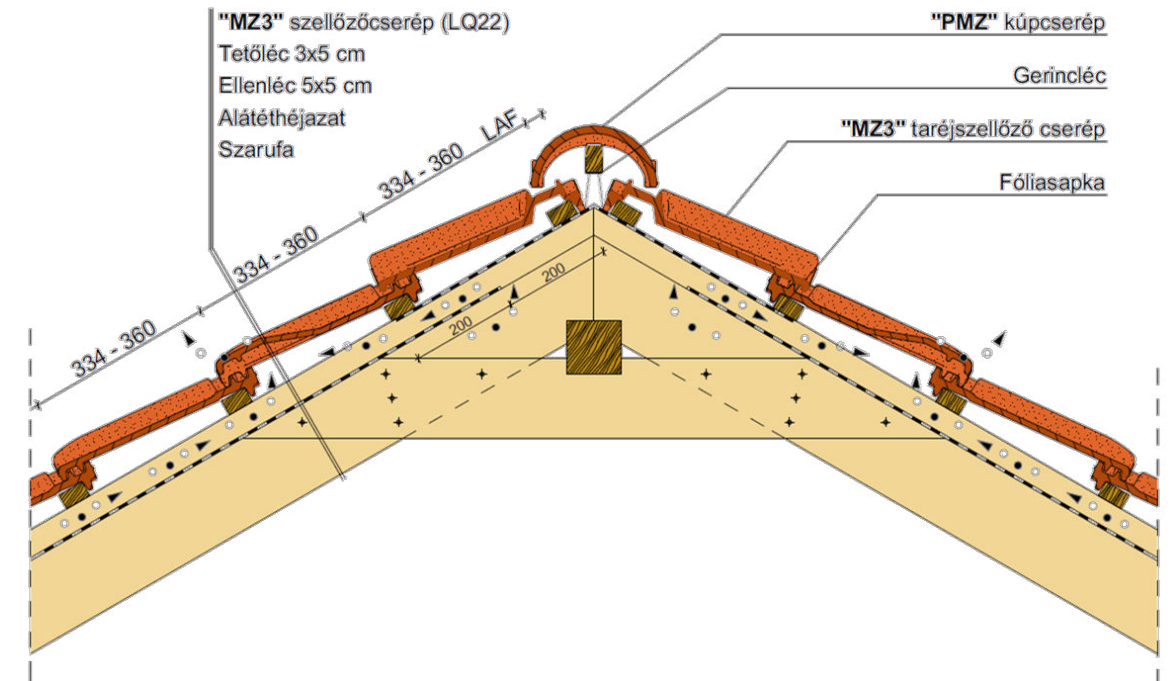
Gerinckialakítás, szellőzőcseréppel
