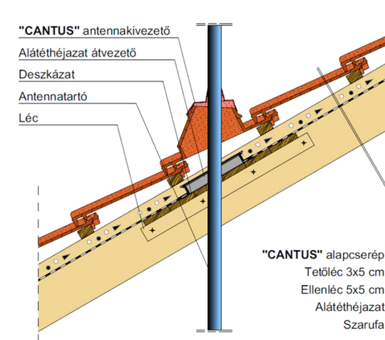
Kerámia antenna átvezetés
