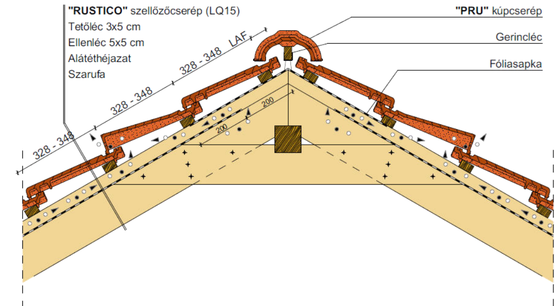
Gerinckialakítás, szellőzőcseréppel
