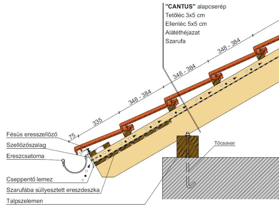
Ereszkialakítás
