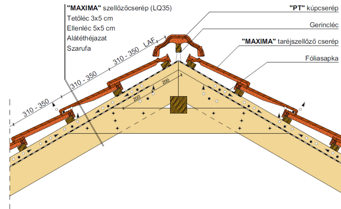
Gerinckialakítás, szellőzőcseréppel
