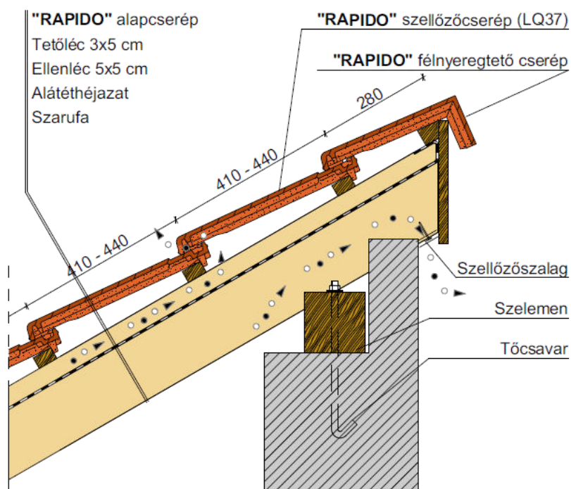
Félnyereggtető gerinc, félnyereggtető cseréppel
