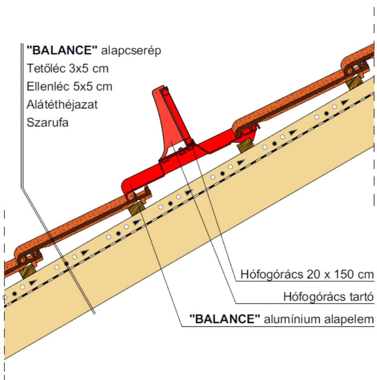
Hófogórács elhelyezése
