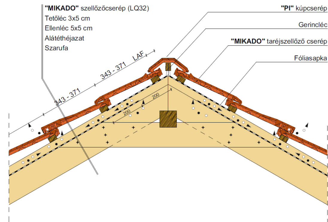
Gerinckialakítás, szellőzőcseréppel
