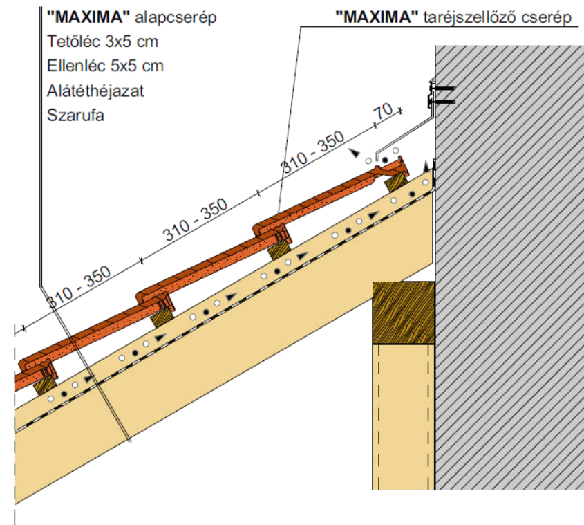
Falszegély kialakítás
