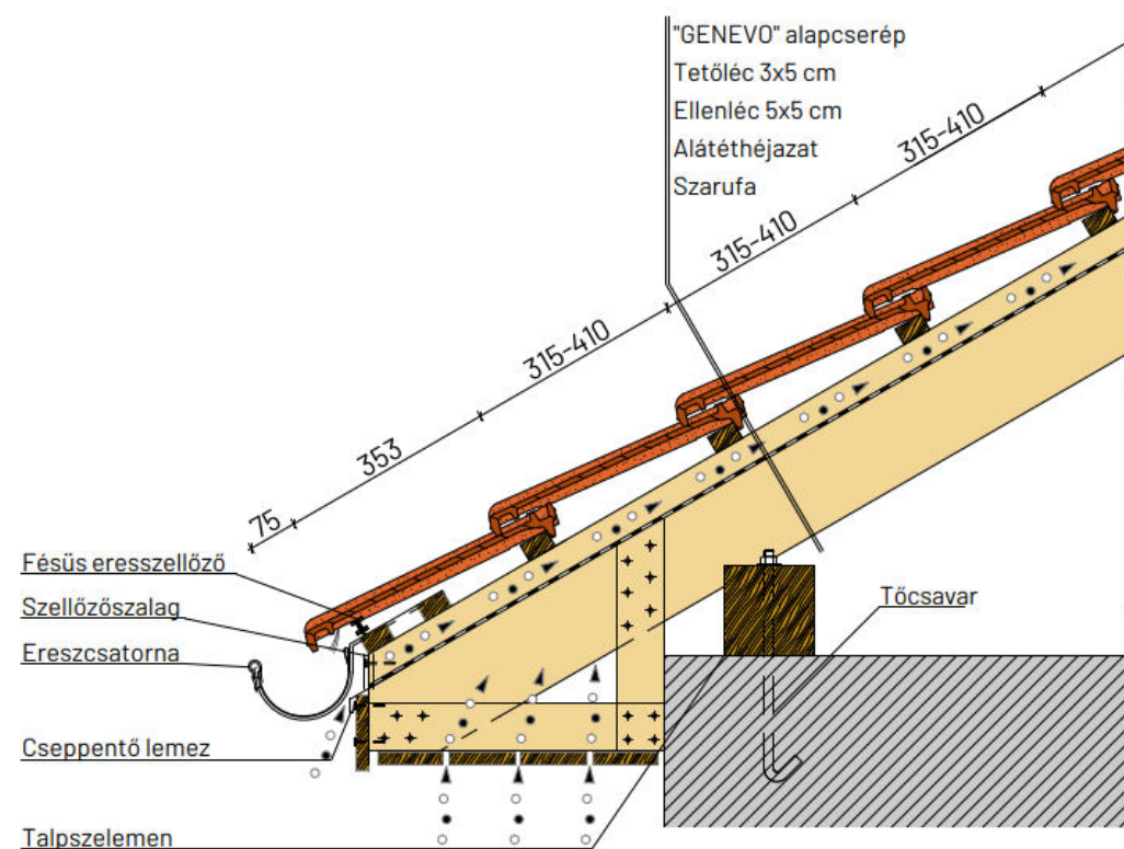
Dobozt ereszkialakítás
