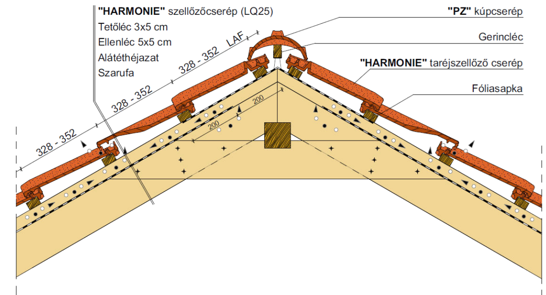
Gerinckialakítás, szellőzőcseréppel
