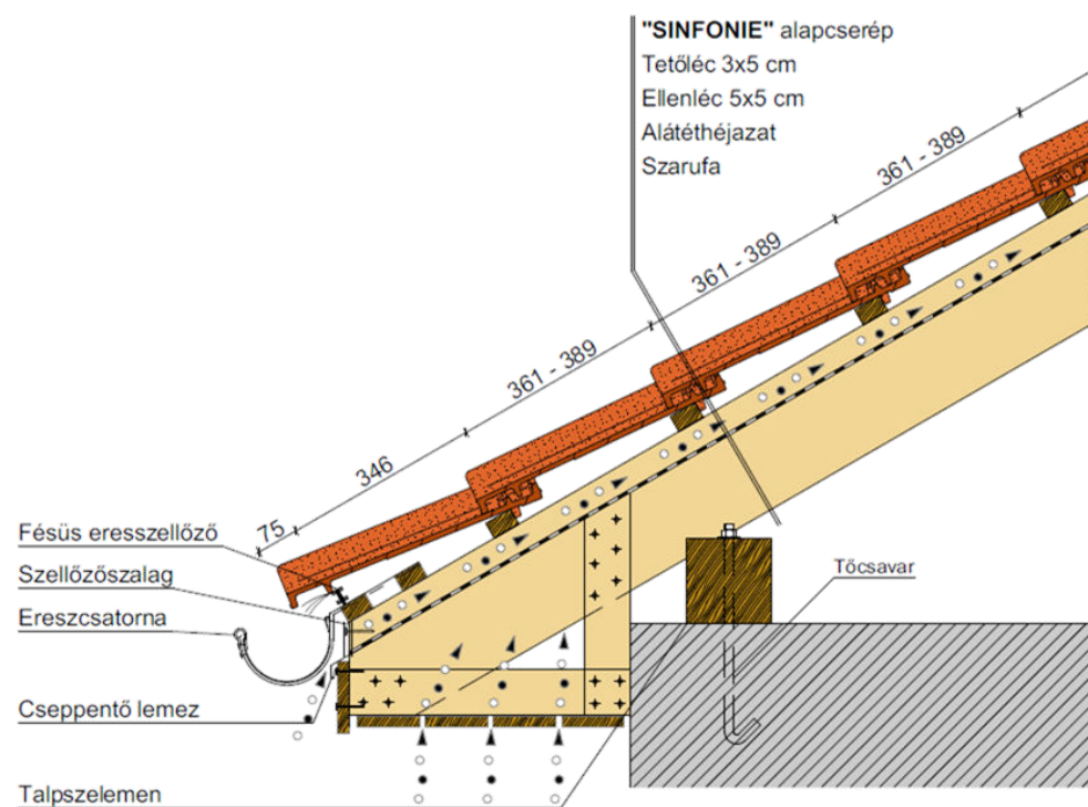
Dobozolt ereszkialakítás
