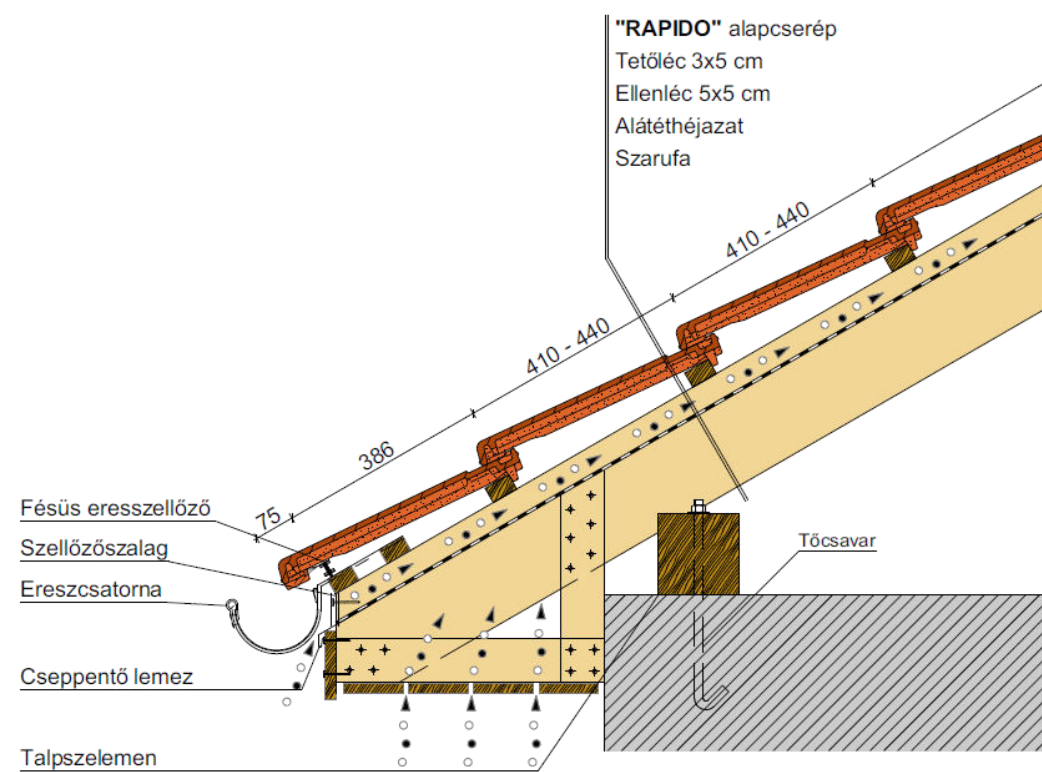
Dobozolt ereszkialakítás
