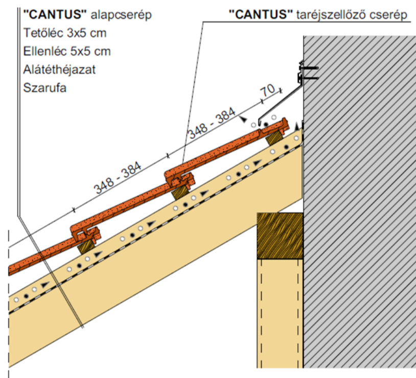
Falszegély kialakítás
