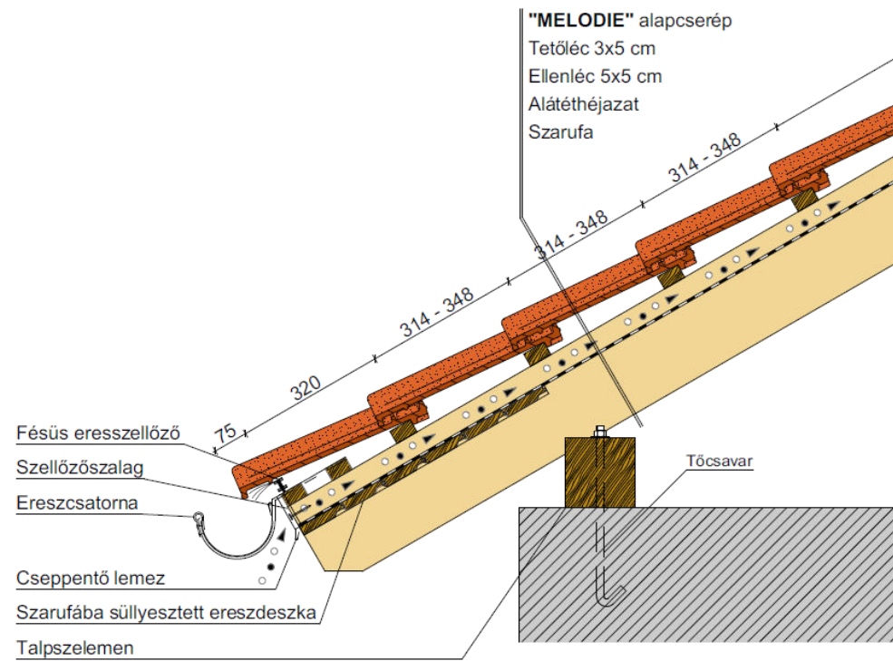
Ereszkialakítás
