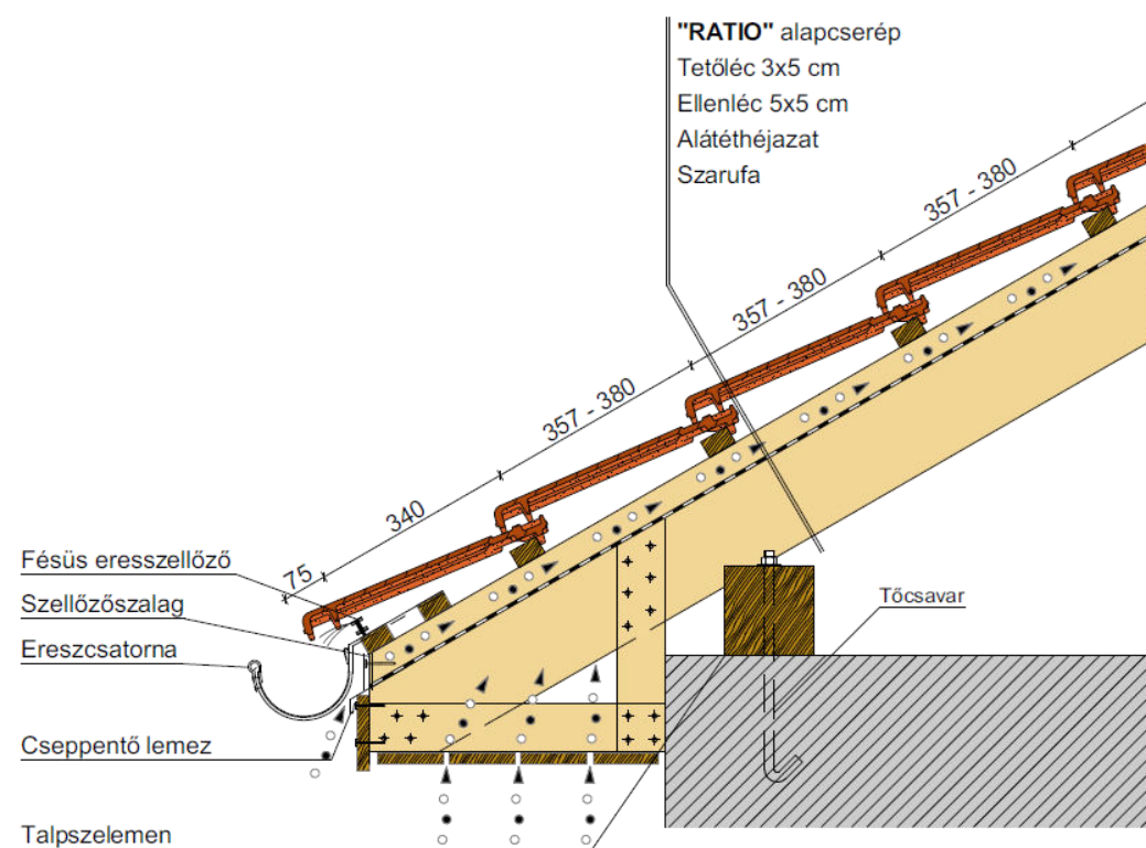
Dobozolt ereszkialakítás
