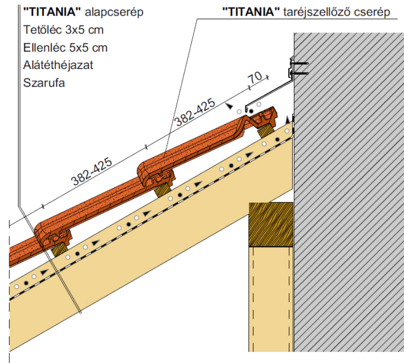
Falszegély kialakítás
