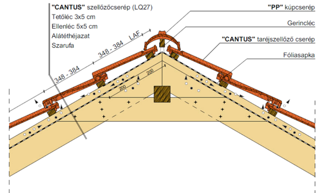
Gerinckialakítás, szellőzőcseréppel
