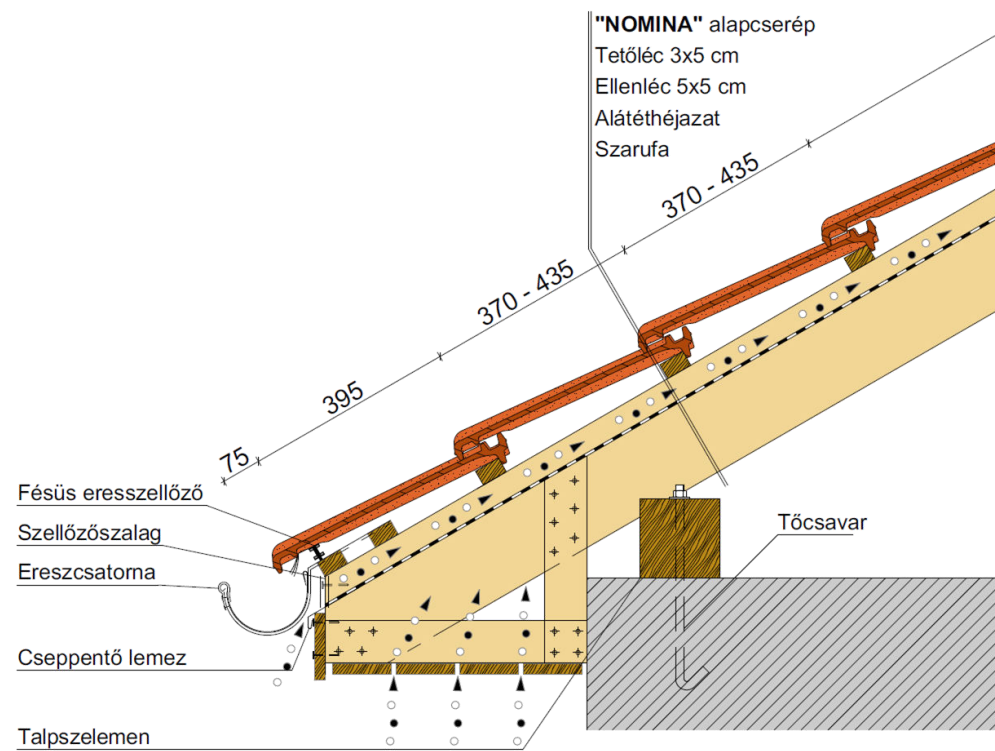
Dobozolt ereszkialakítás
