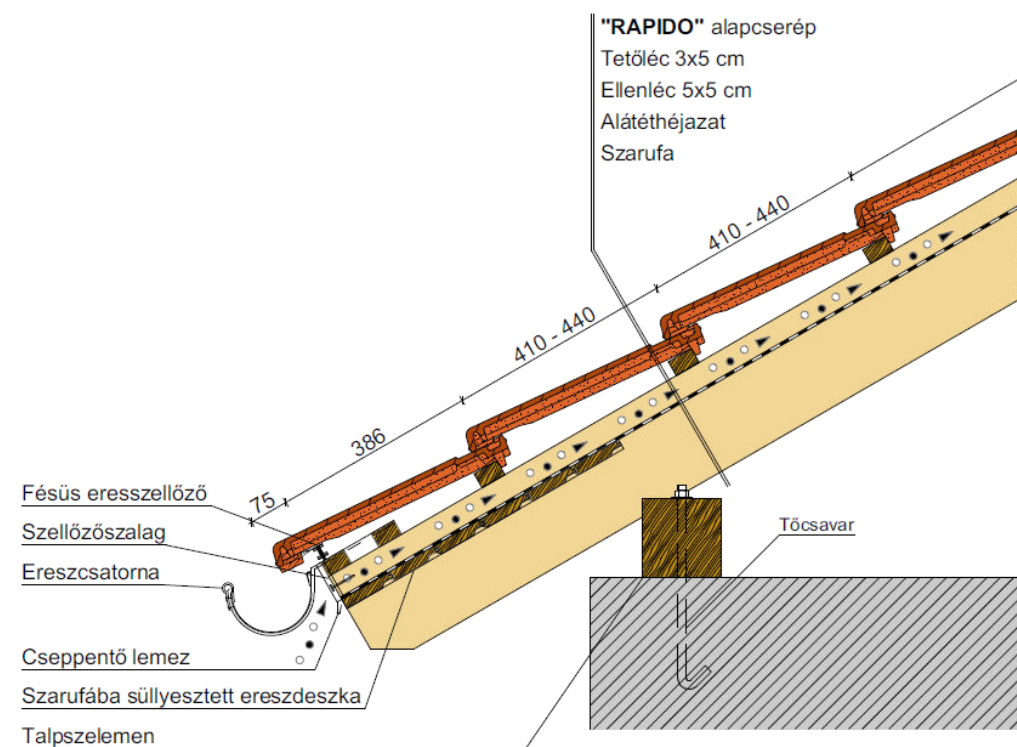
Ereszkialakítás
