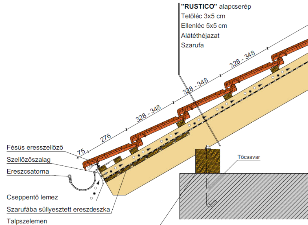
Ereszkialakítás
