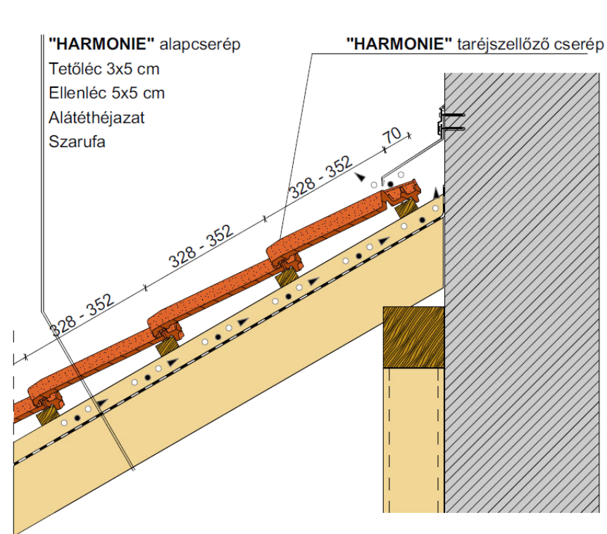
Falszegély kialakítás
