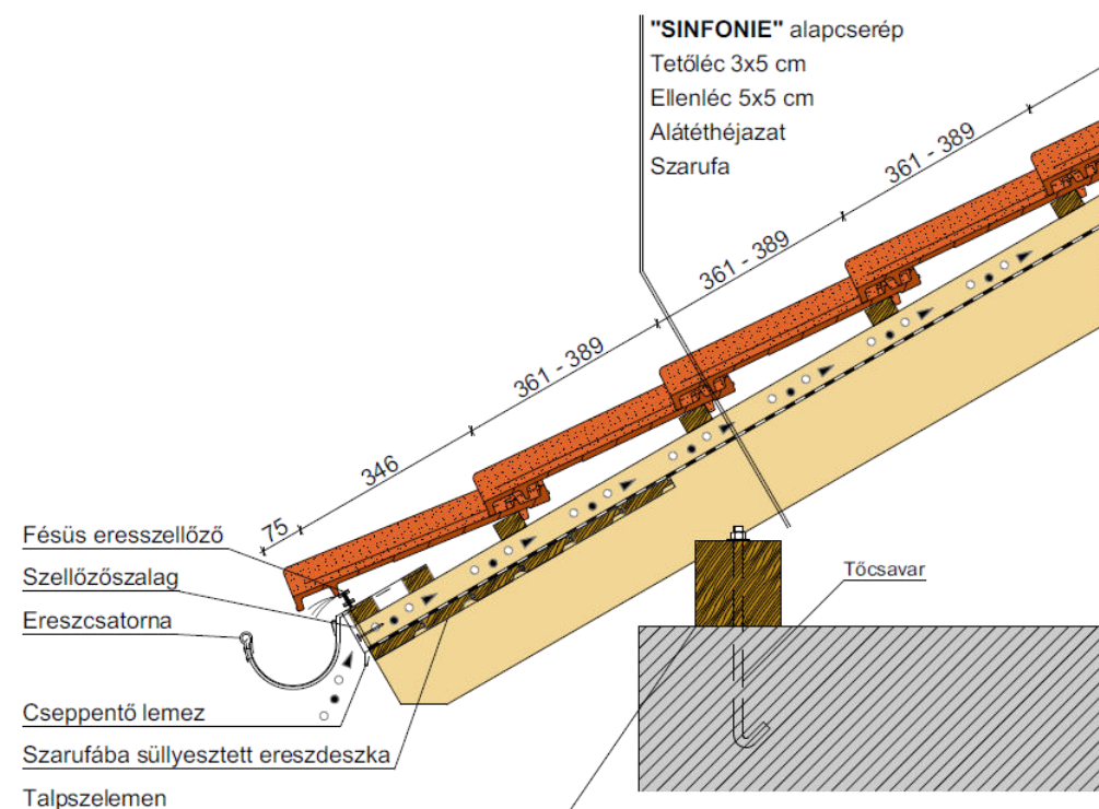
Ereszkialakítás
