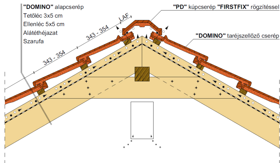
Gerinckialakítás, taréjszellőző cseréppel
