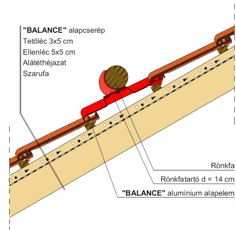
Rönkfartató elhelyezése
