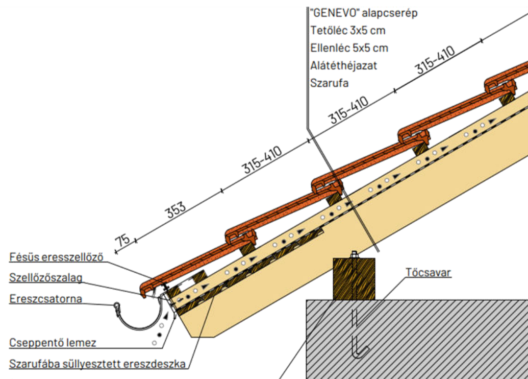
Ereszkialakítás
