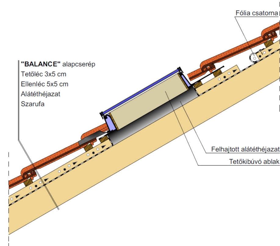
Tetőkibúvó ablak elhelyezése
