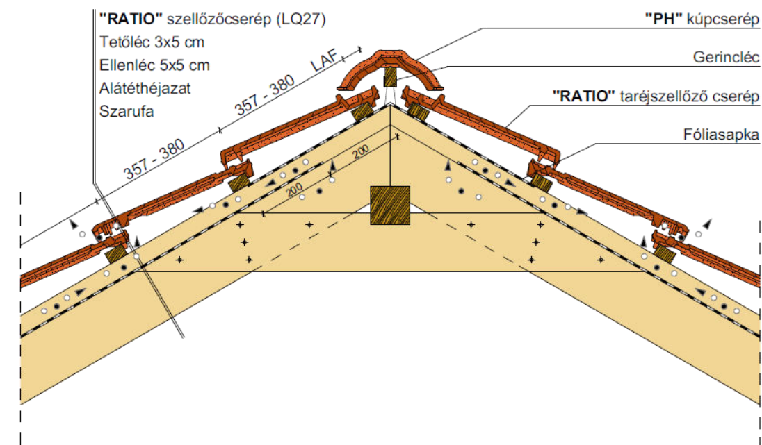
Gerinckialakítás, szellőzőcseréppel
