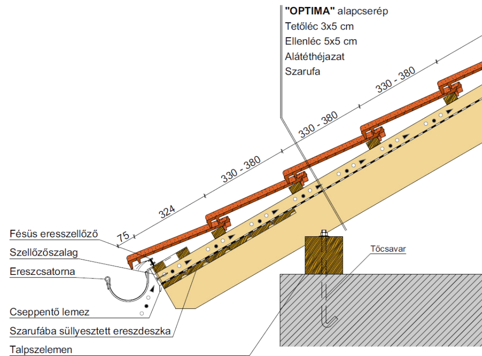
Ereszkialakítás
