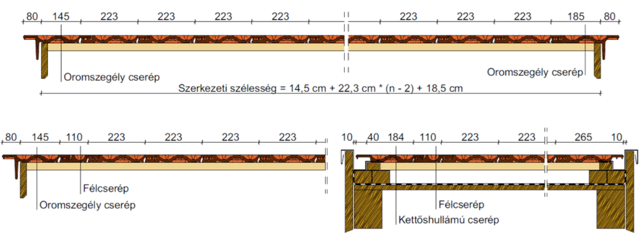
Fedési szélesség oromdeszkától-oromdeszkáig
