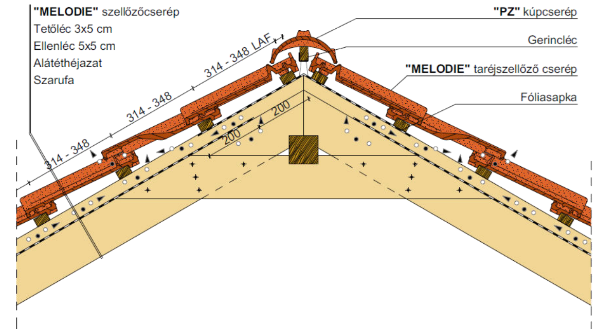
Gerinckialakítás, szellőzőcseréppel
