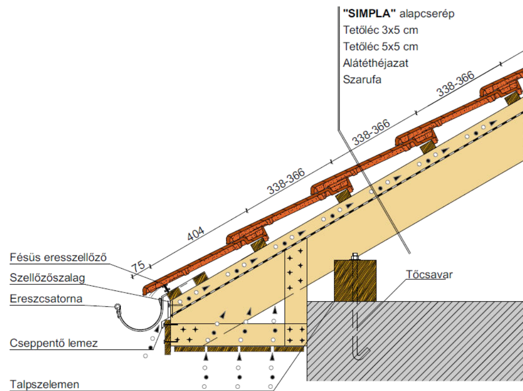
Dobozolt ereszkialakítás
