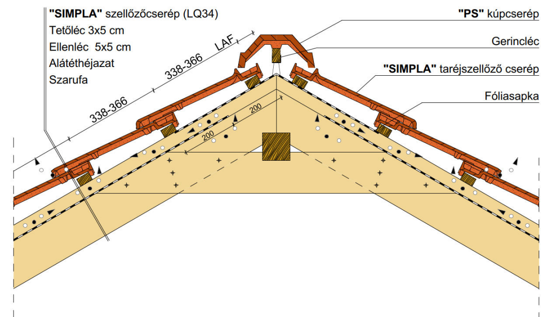
Gerinckialakítás, szellőzőcseréppel
