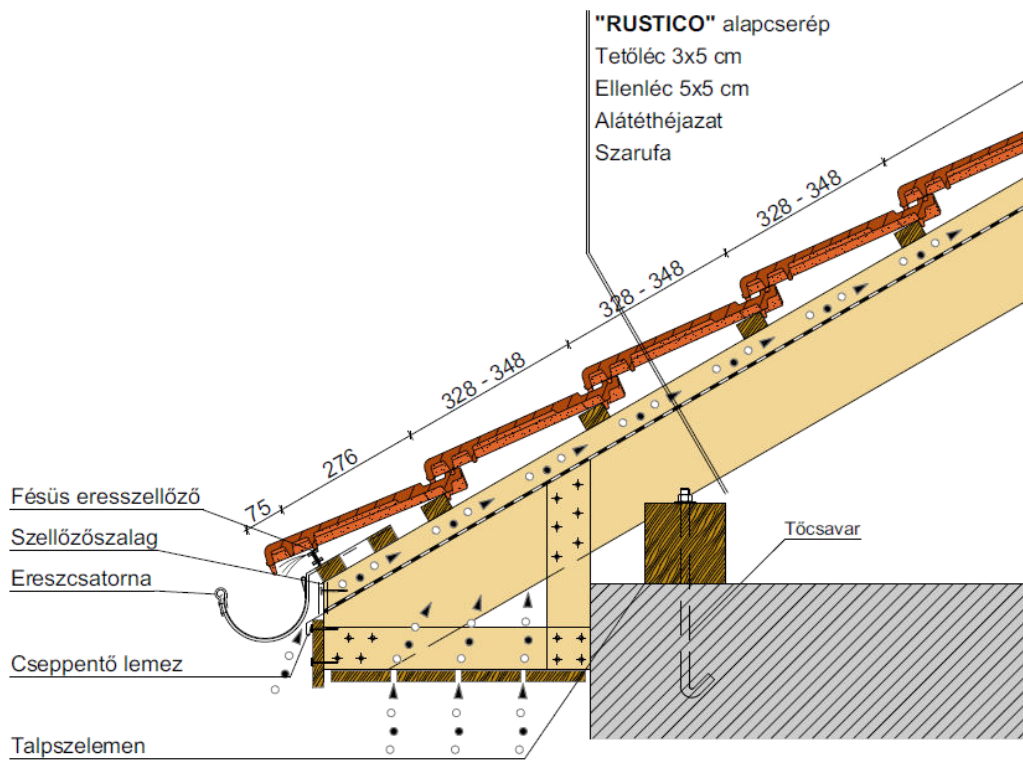
Dobozolt ereszkialakítás
