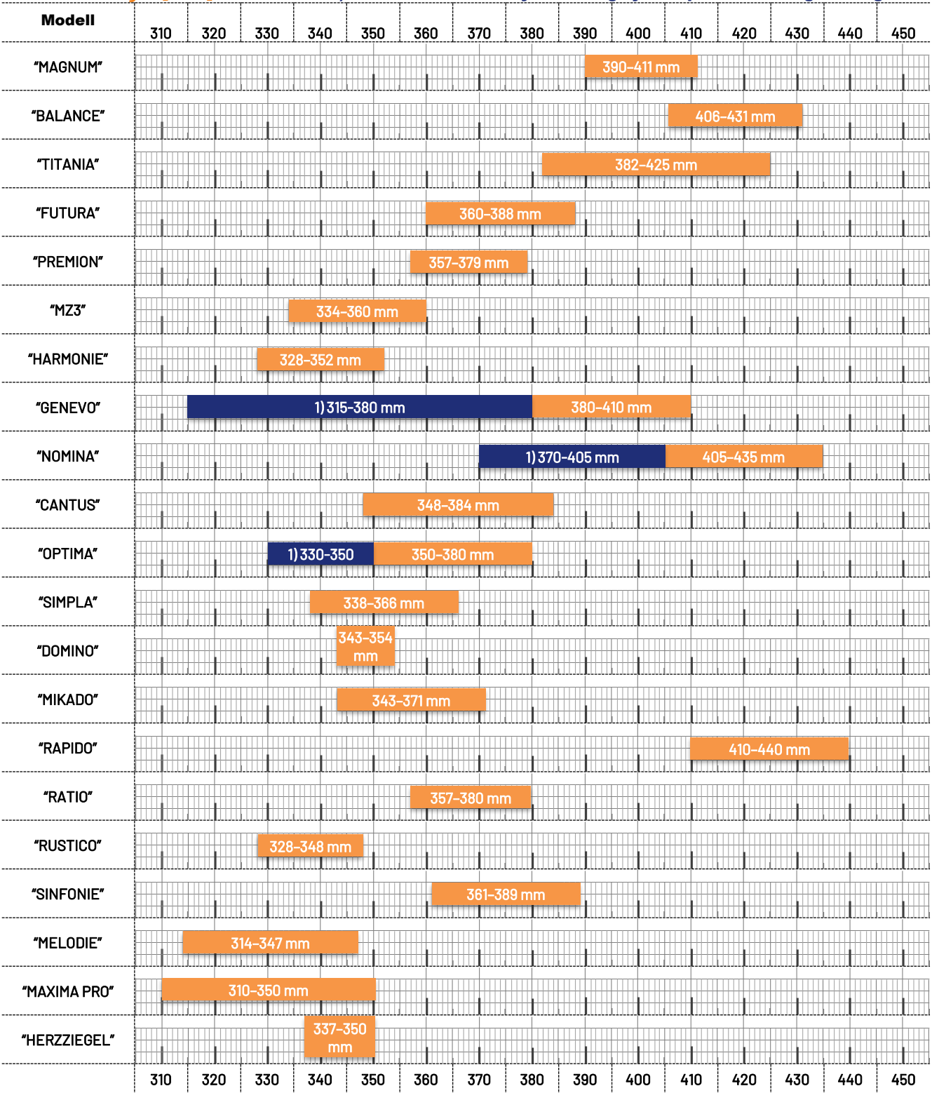
Léctávolságok [mm] áttekintése 1.) Az ábrázolt tartományban a szegélycserepek sarkát meg kell vágni!
