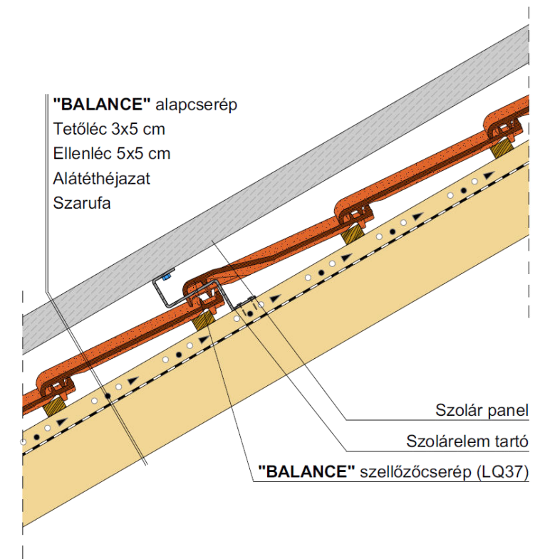
Szolárelem tartó szett elhelyezése
