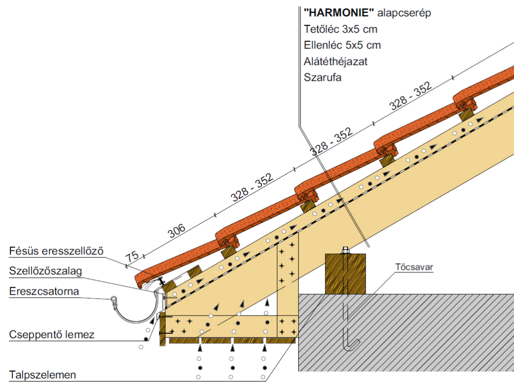
Dobozolt ereszkialakítás
