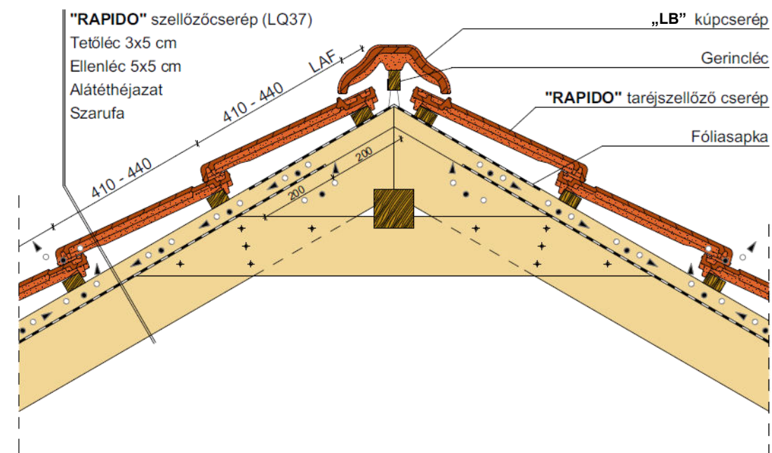
Gerinckialakítás, szellőzőcseréppel
