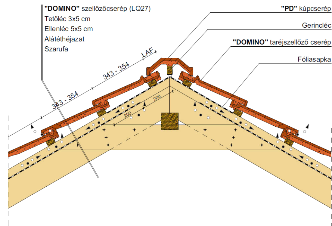
Gerinckialakítás, szellőzőcseréppel
