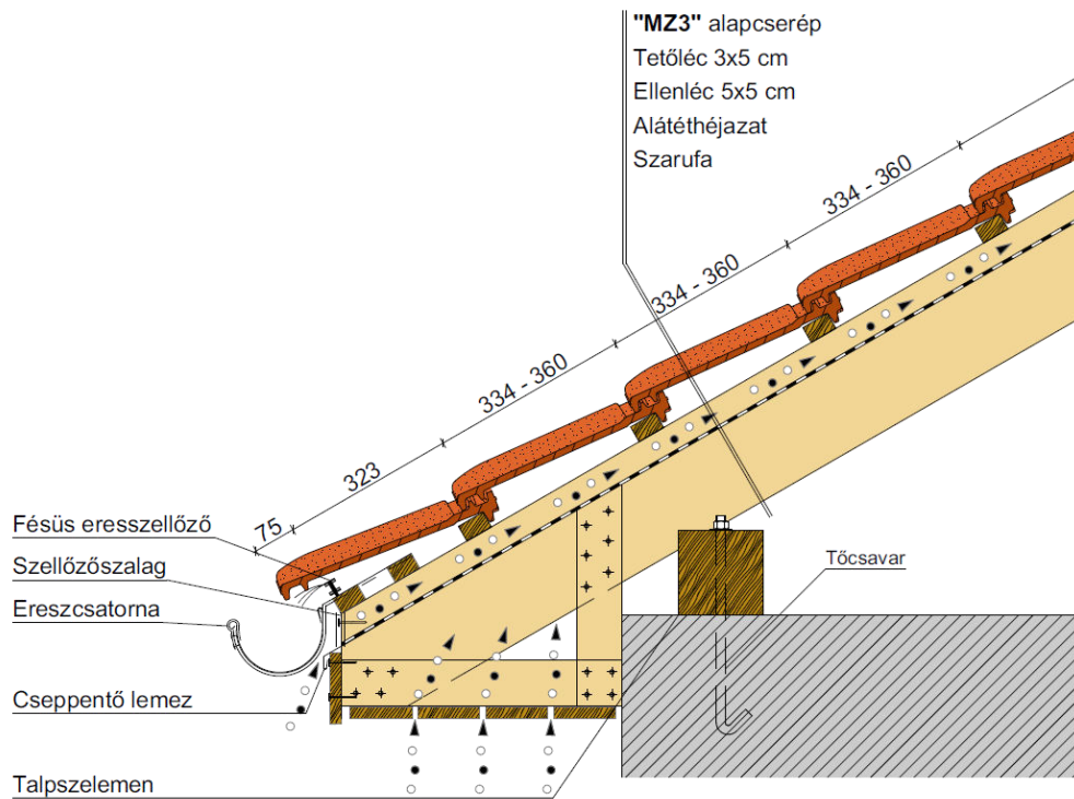
Dobozolt ereszkialakítás
