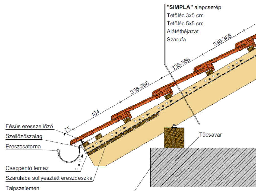
Ereszkialakítás
