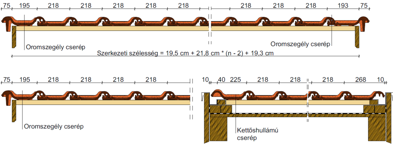
Fedési szélesség oromdeszktól-oromdeszkáig
