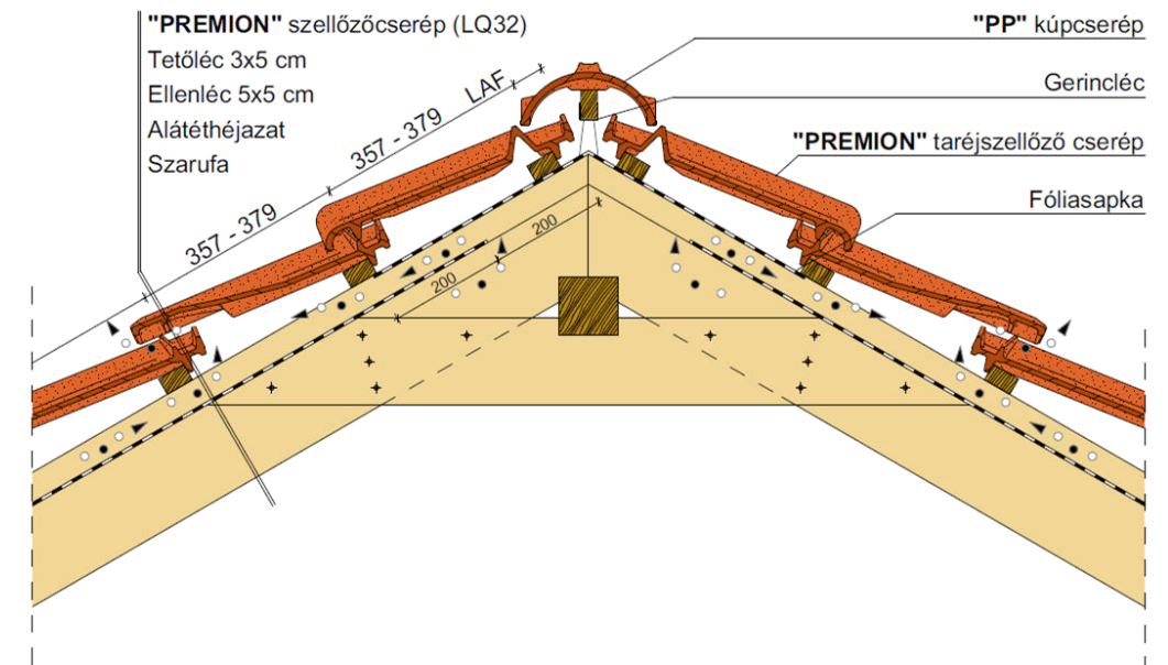
Gerinckialakítás, szellőzőcseréppel
