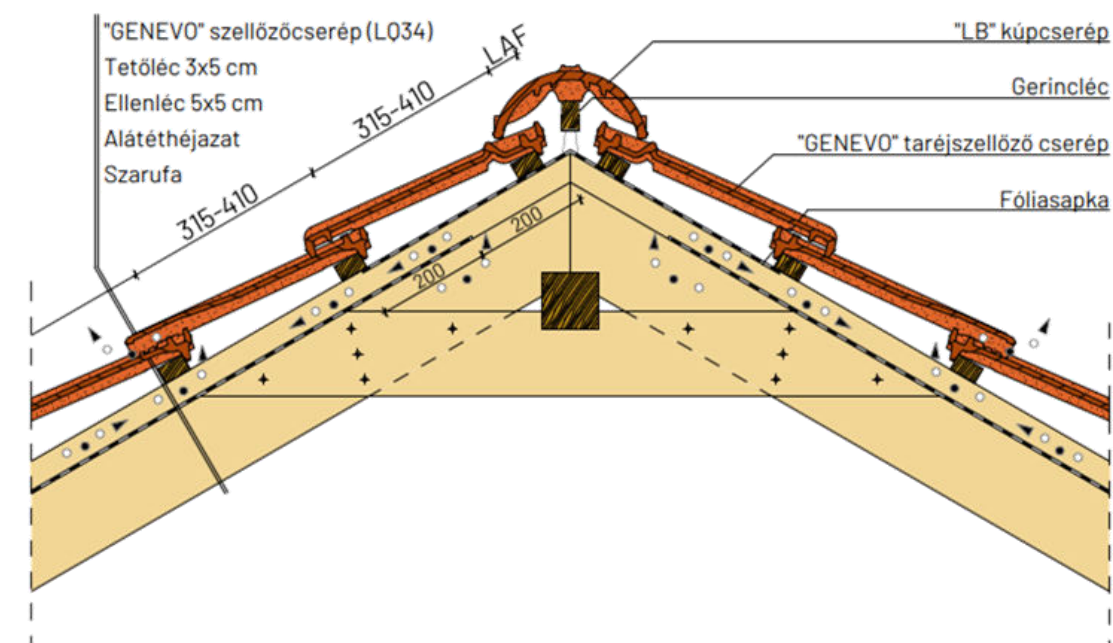
Gerinckialakítás, szellőzőcseréppel
