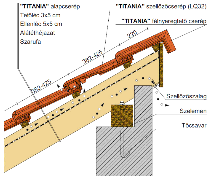
Félnyeregvető gerinc, félnyeregvető cseréppel
