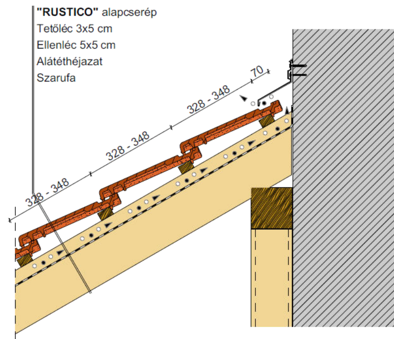
Falszegély kialakítás
