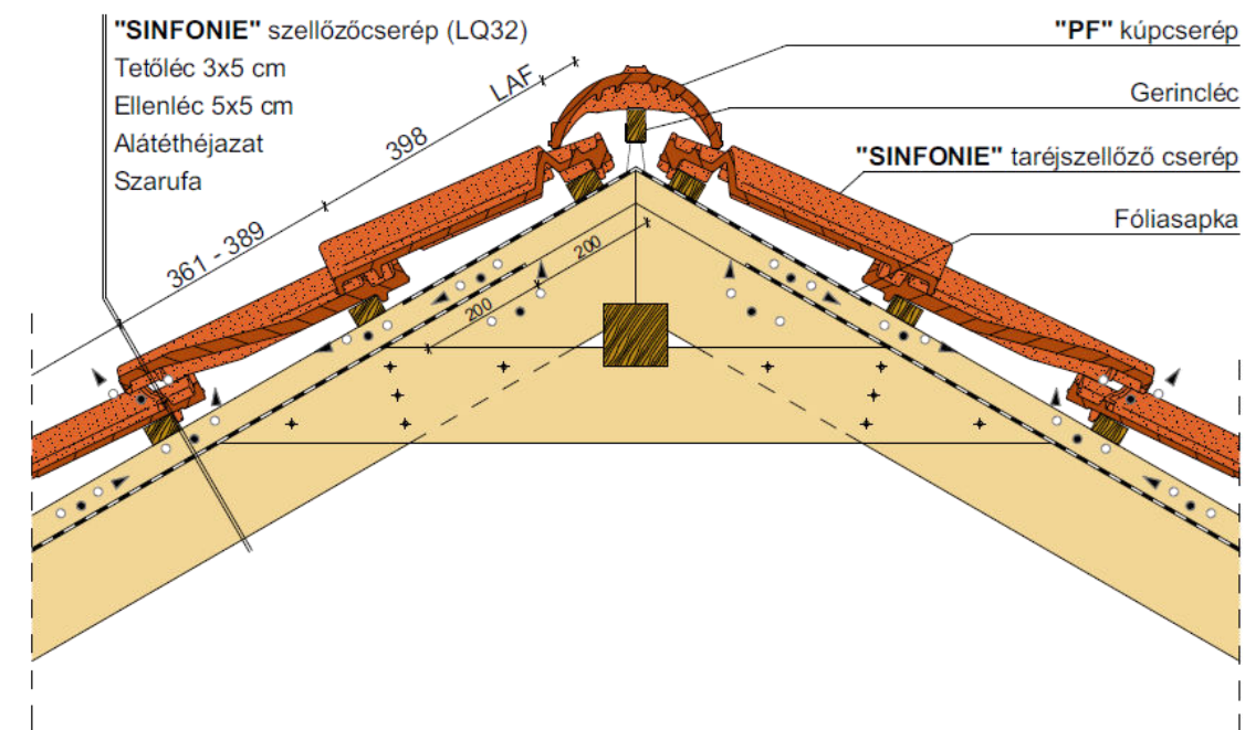
Gerinckialakítás, szellőzőcseréppel
