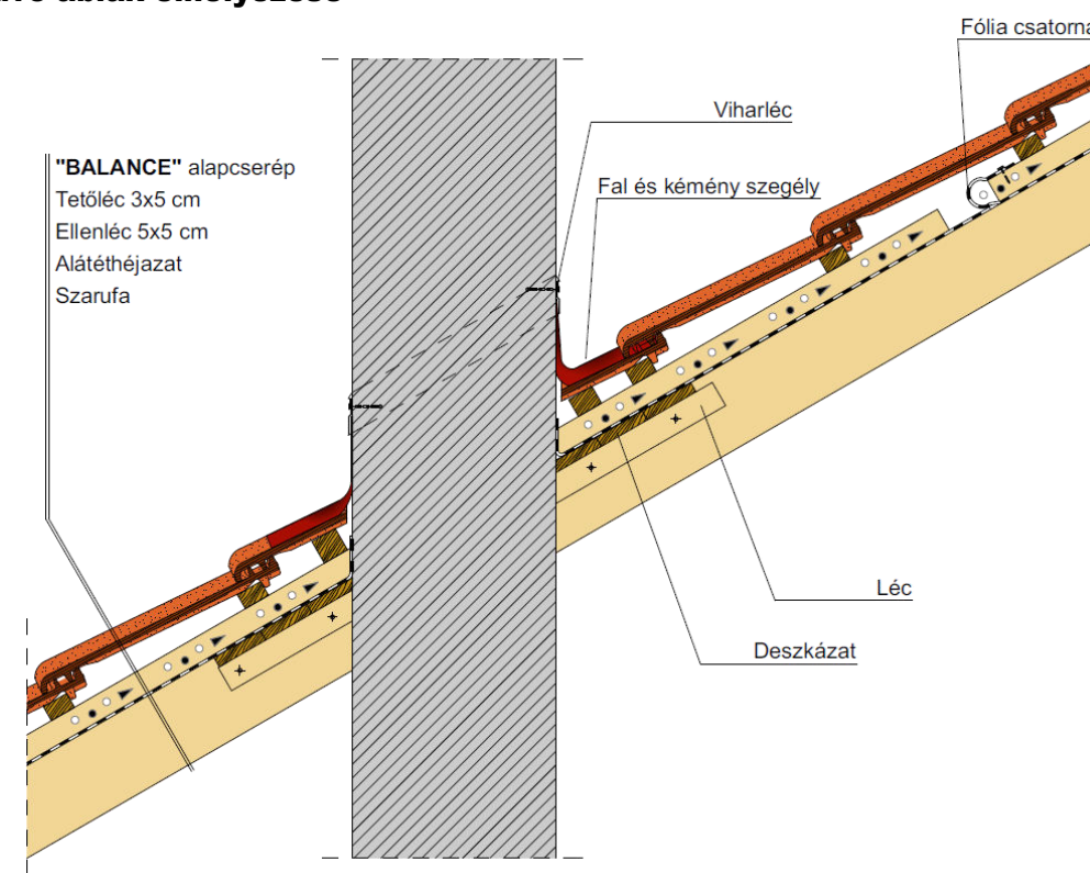
Kéményszegély kialakítása
