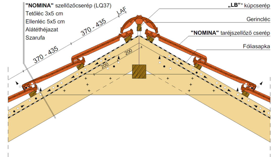
Gerinckialakítás, szellőzőcseréppel
