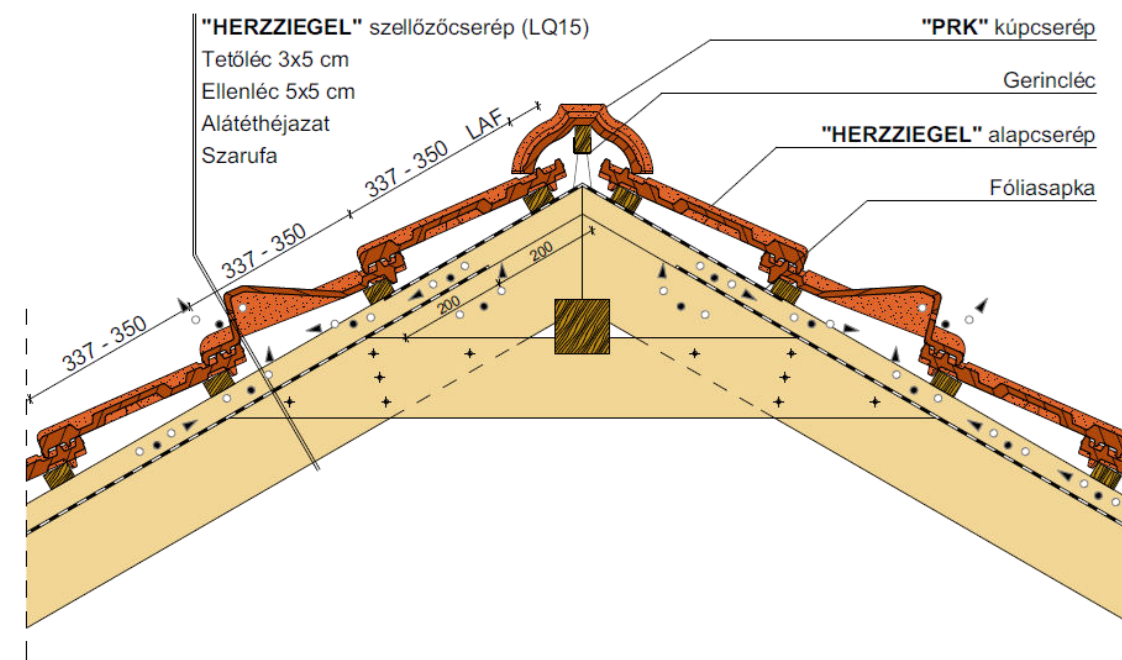
Gerinckialakítás, szellőzőcseréppel
