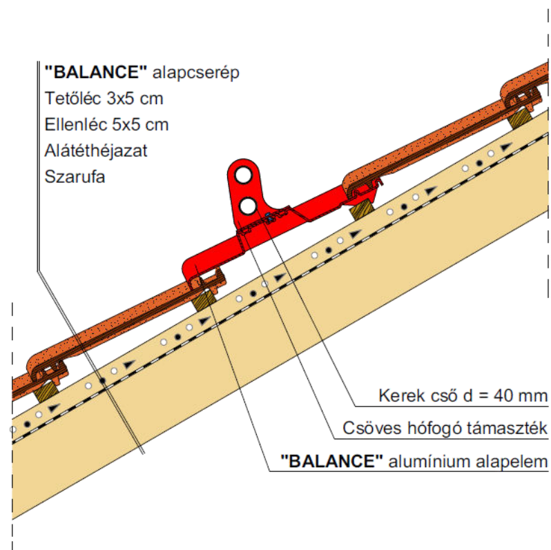
Hófogócső elhelyezése
