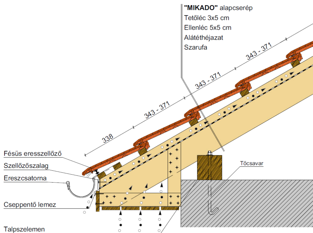
Dobozolt ereszkialakítás
