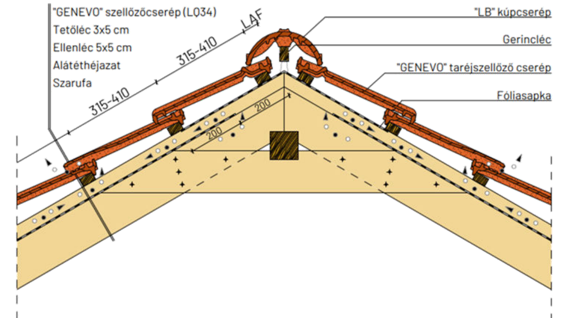
Gerinckialakítás, szellőzőcseréppel
