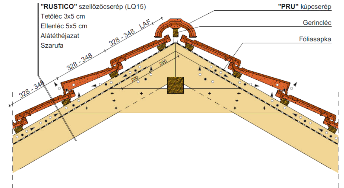
Gerinckialakítás, szellőzőcseréppel
