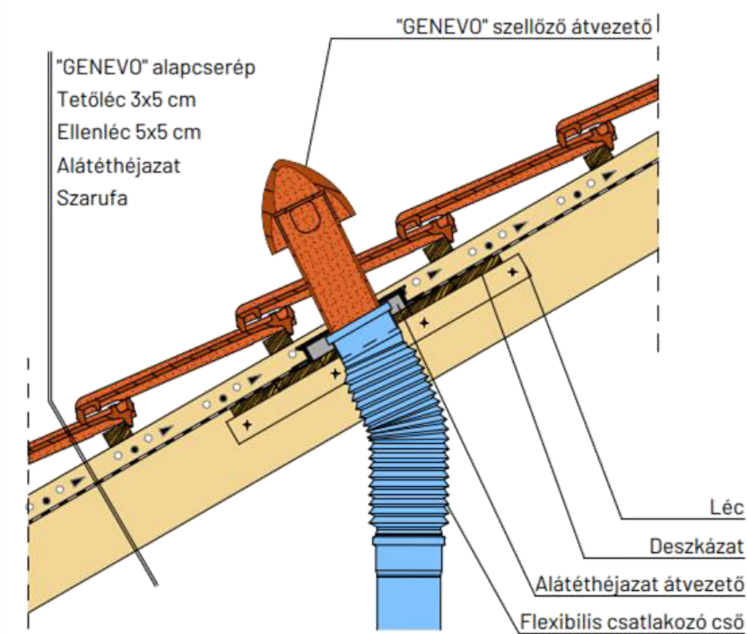
Kerámia csatornaszellőző átvetése
