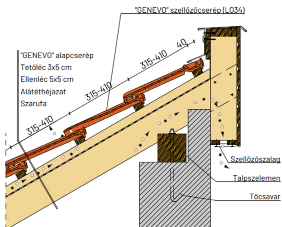
Félnyeregű gerinc, félnyeregű cseréppel
