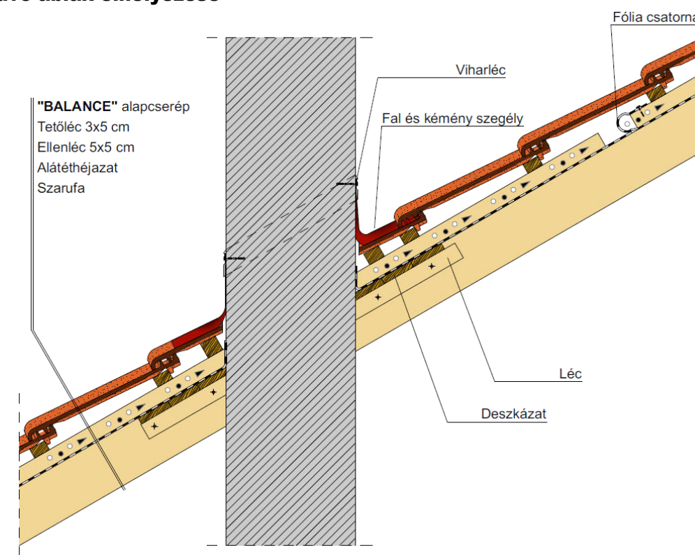
Kéményszegély kialakítása
