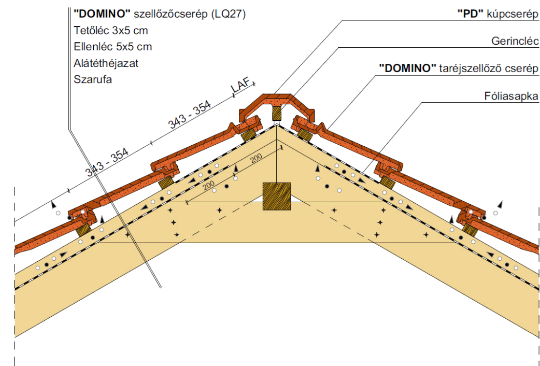
Gerinckialakítás, szellőzőcseréppel
