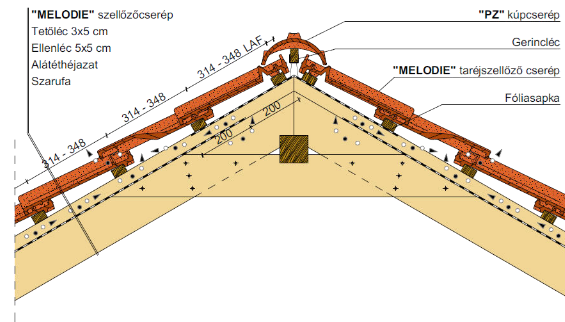
Gerinckialakítás, szellőzőcseréppel
