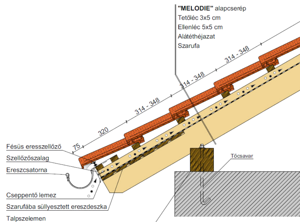
Ereszkialakítás
