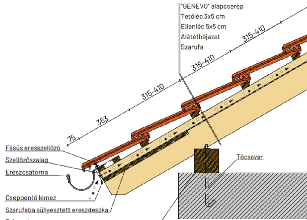
Ereszkialakítás
