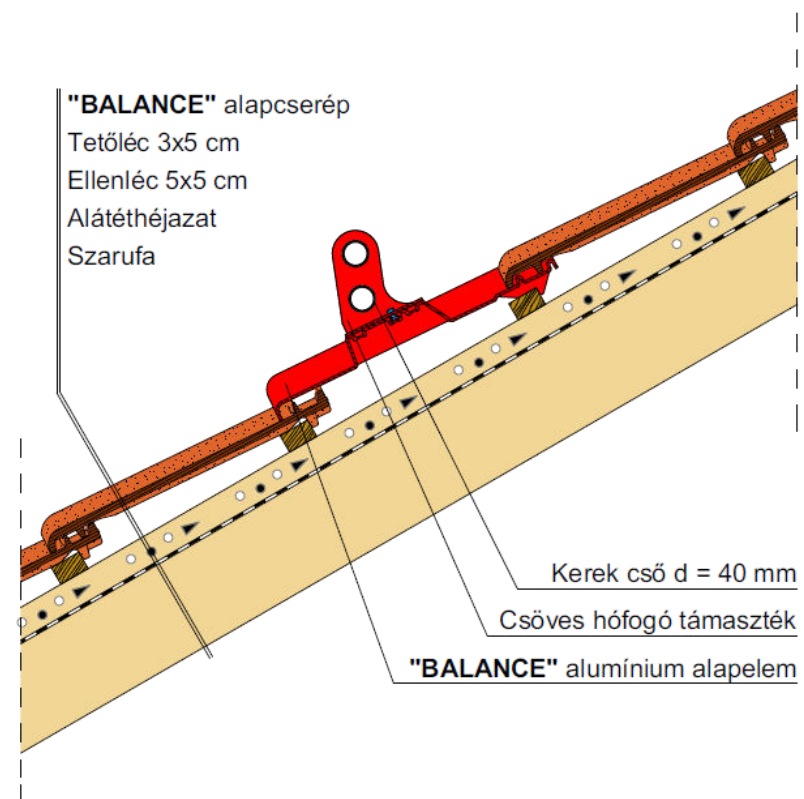
Hófogócső elhelyezése
