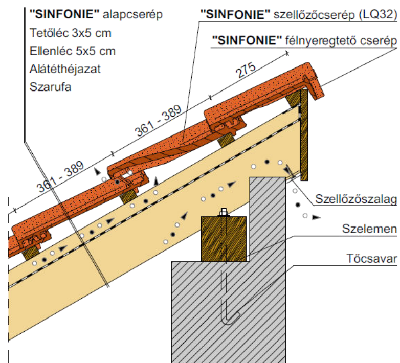
Félnyereggető gerinc, félnyereggető cseréppel
