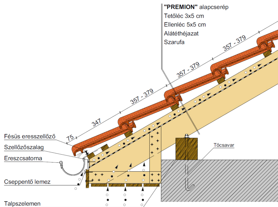
Dobozt ereszkialakítás
