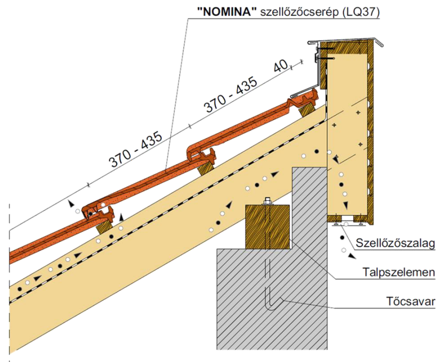
Félnyeregűtető gerinc, félnyeregűtető cseréppel
