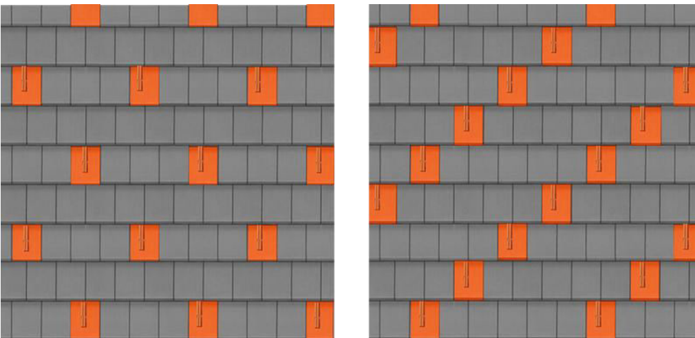
swissporTON NIVELLO, 9,8 db/m 2 anyagigénnyel
