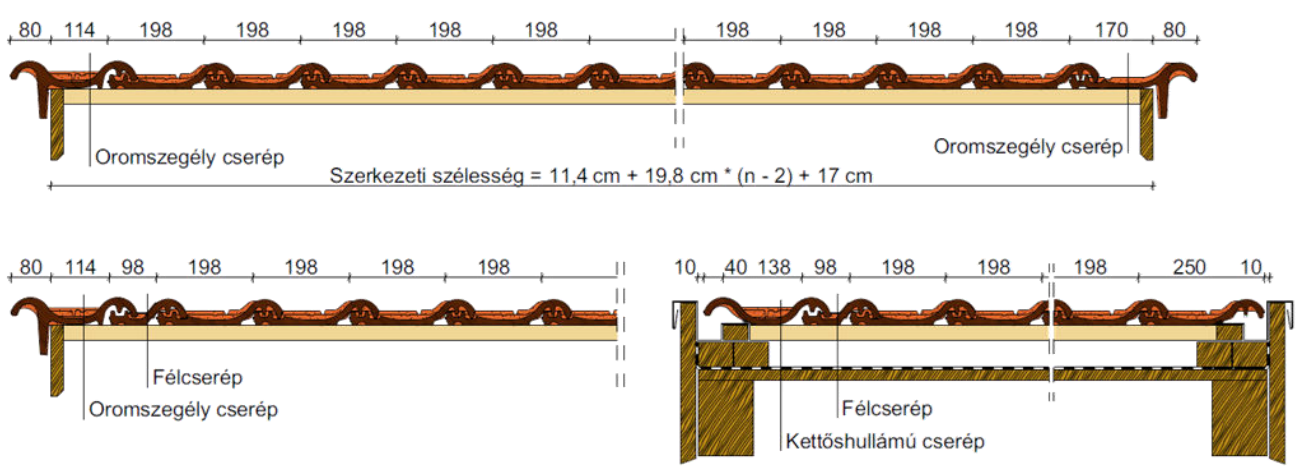
Fedési szélesség oromdeszktól-oromdeszkáig
