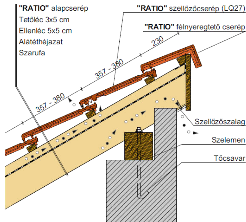
Félnyeregvető gerinc, félnyeregvető cseréppel
