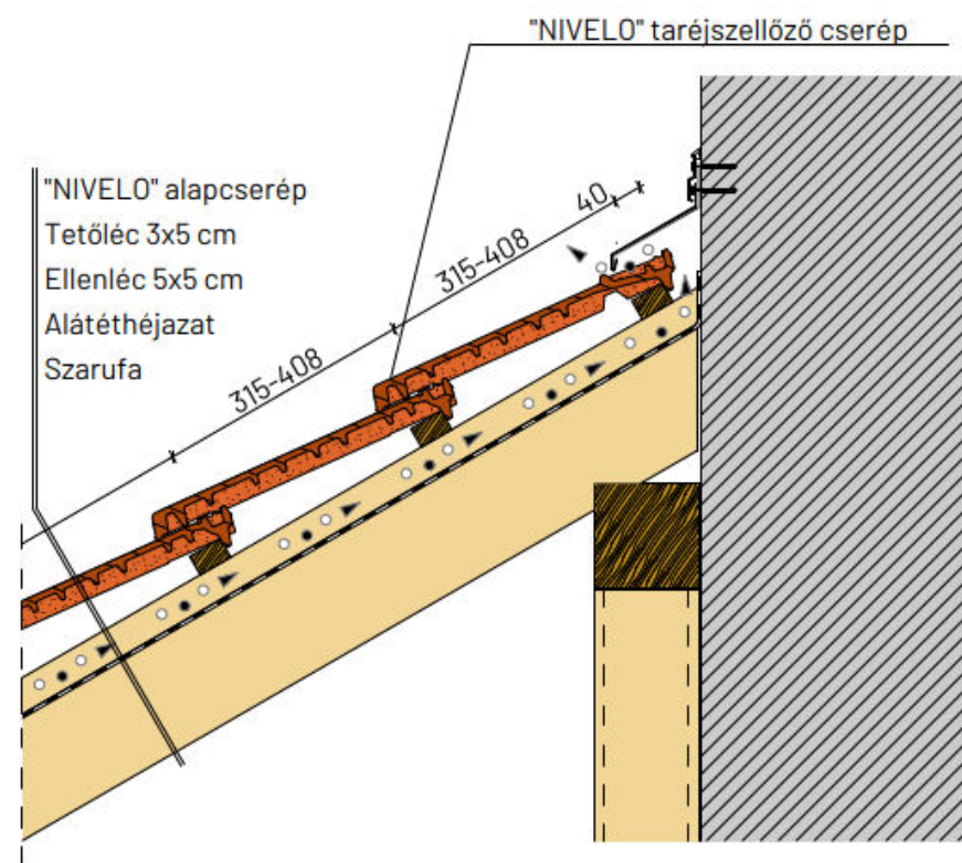
Falszegély kialakítás
