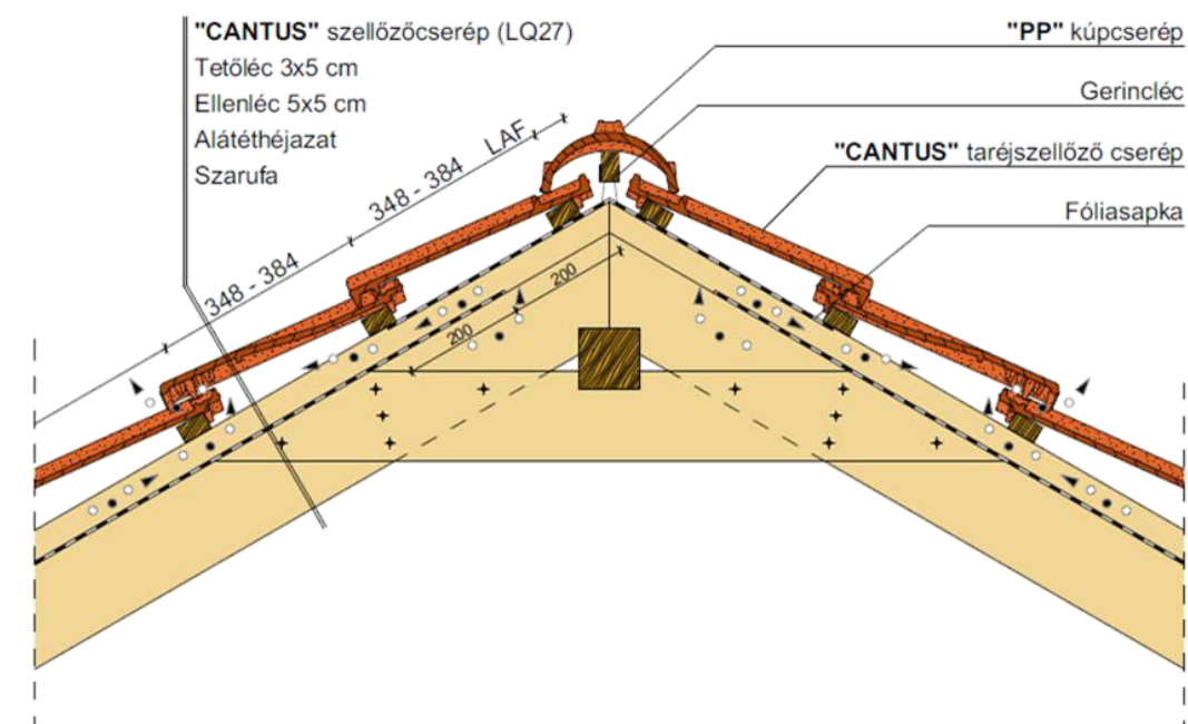
Gerinckialakítás, szellőzőcseréppel
