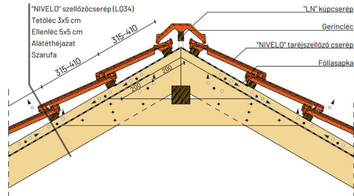
Gerinckialakítás, szellőzőcseréppel
