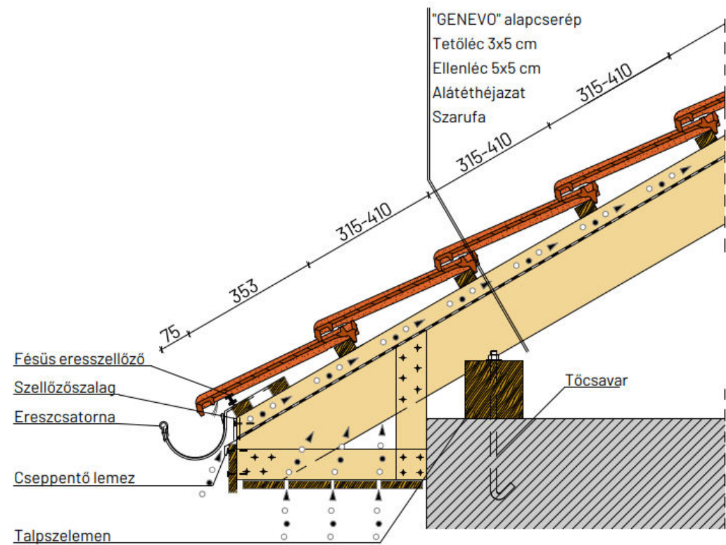
Dobozolt ereszkialakítás
