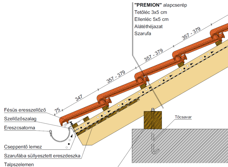
Ereszkialakítás
