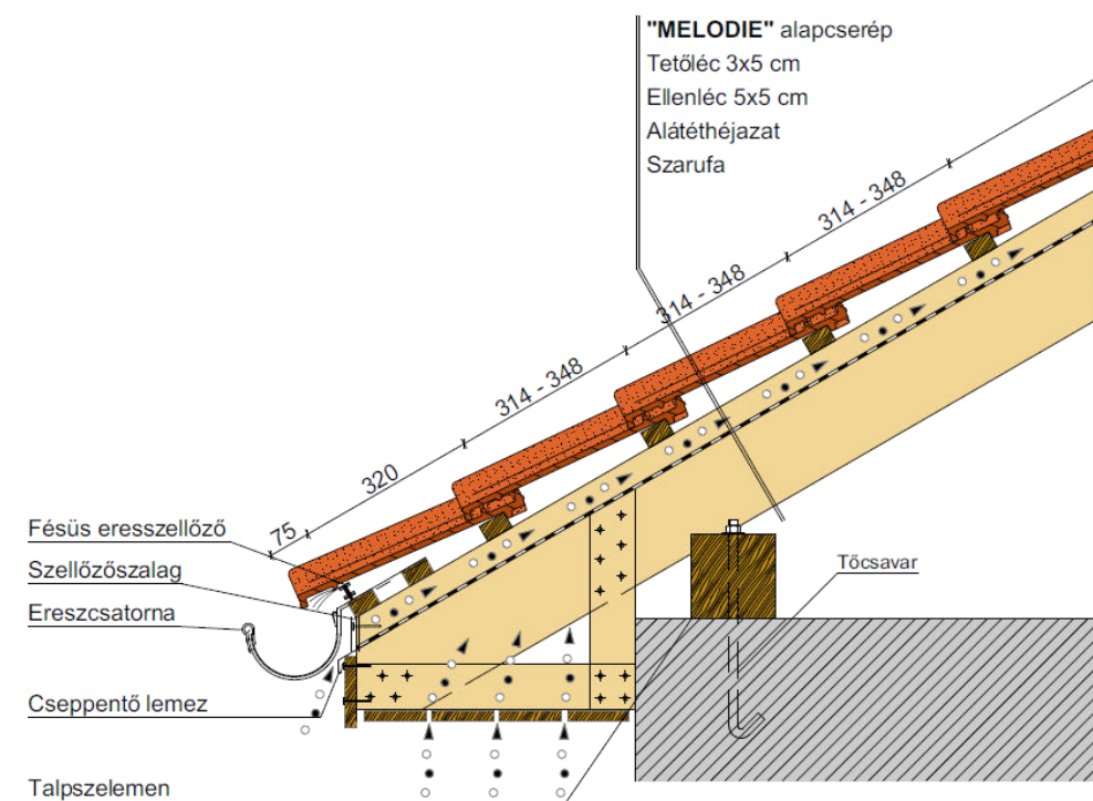
Dobozolt ereszkialakítás
