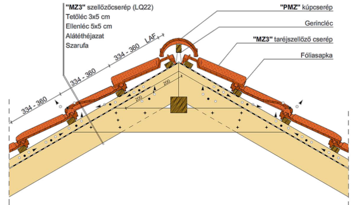
Gerinckialakítás, szellőzőcseréppel
