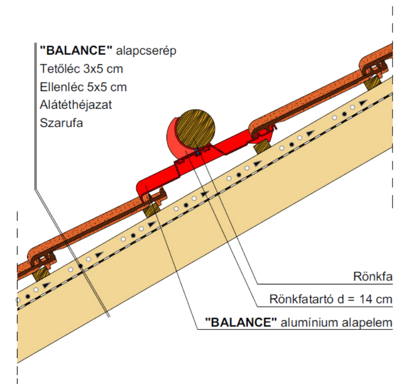
Rönkfartó elhelyezése
