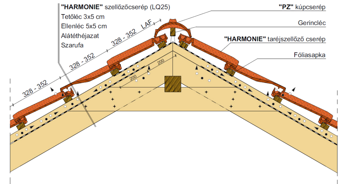
Gerinckialakítás, szellőzőcseréppel
