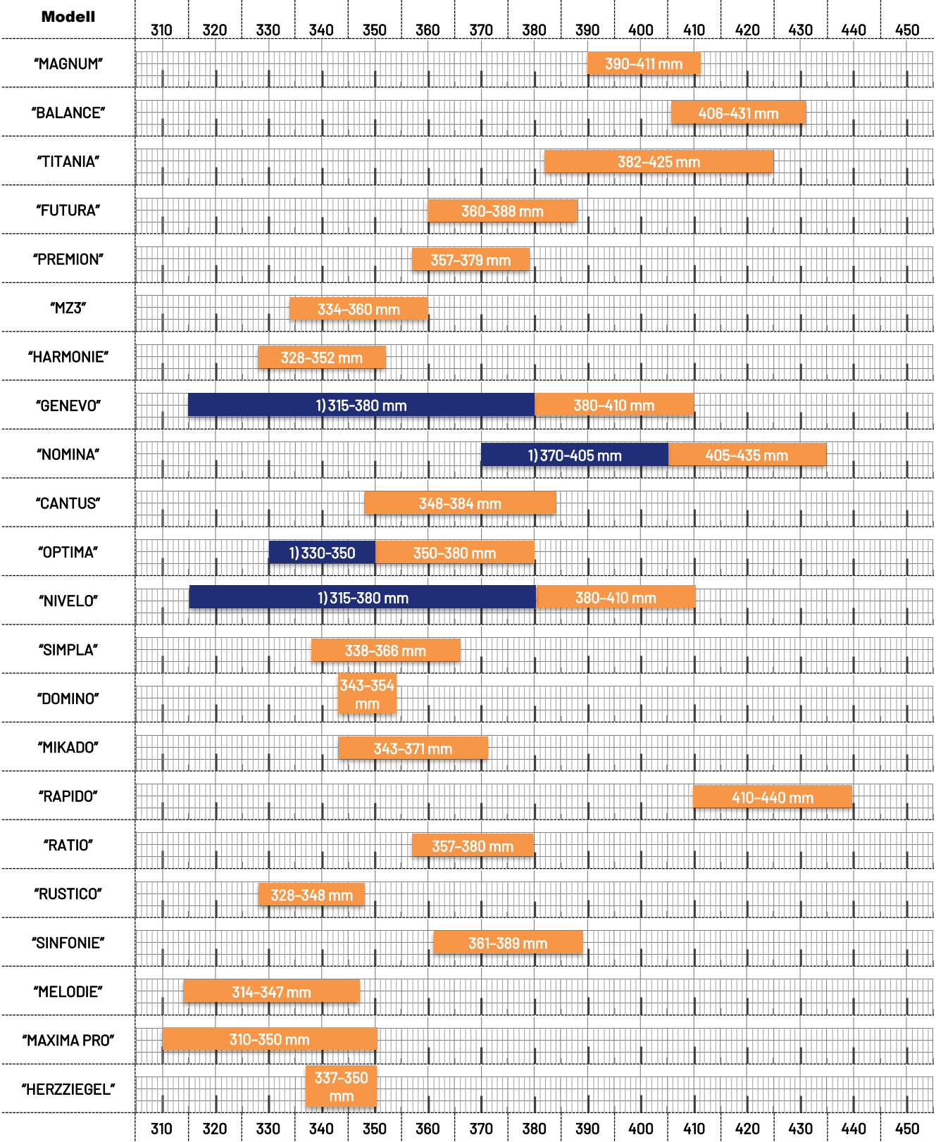
Léctávolságok [mm] áttekintése 1.) Az ábrázolt tartományban a szegélycserepek sarkát meg kell vágni!
