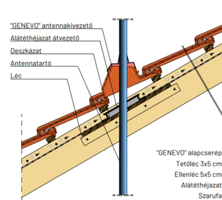
Kerámia antenna átvetése
