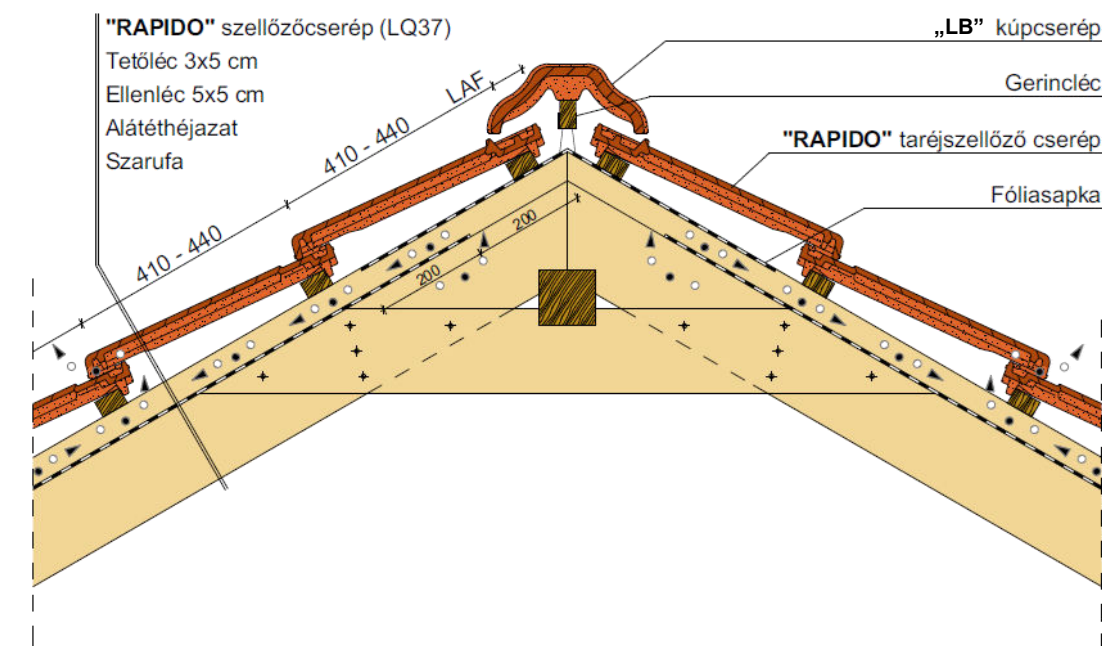
Gerinckialakítás, szellőzőcseréppel
