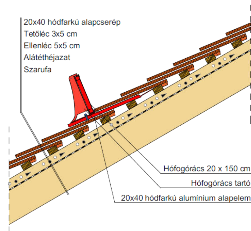
Hófogórács elhelyezése
