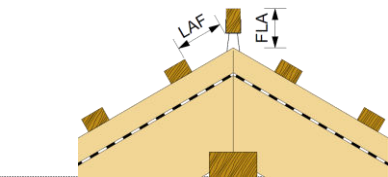
LAF: felső lécs távolsága a gerinccsúcstól
