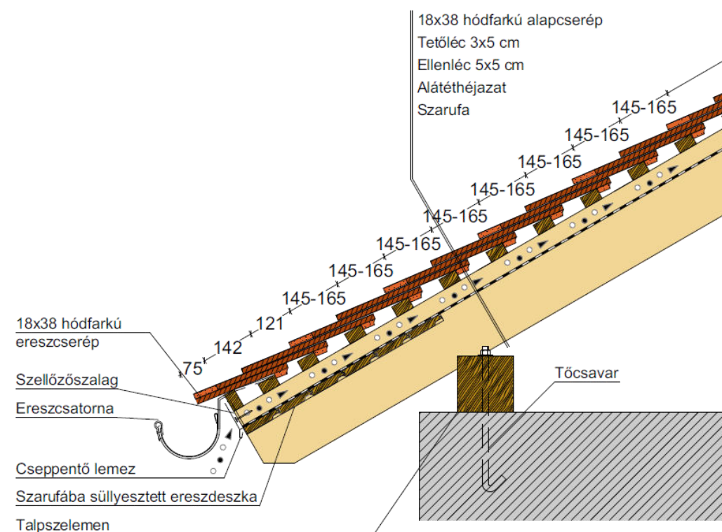
Ereszkialakítás
