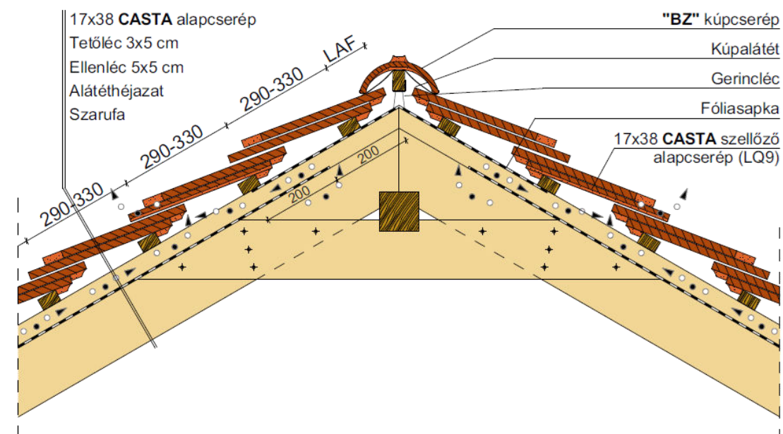
Koronafedésű gerinckialakítás, szellőzőcsereppel,
