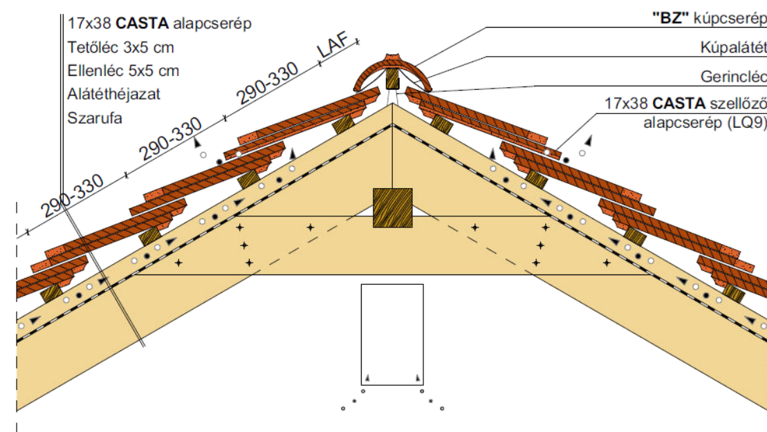
Koronafedésű gerinckialakítás, szellőző alapcsereppel
