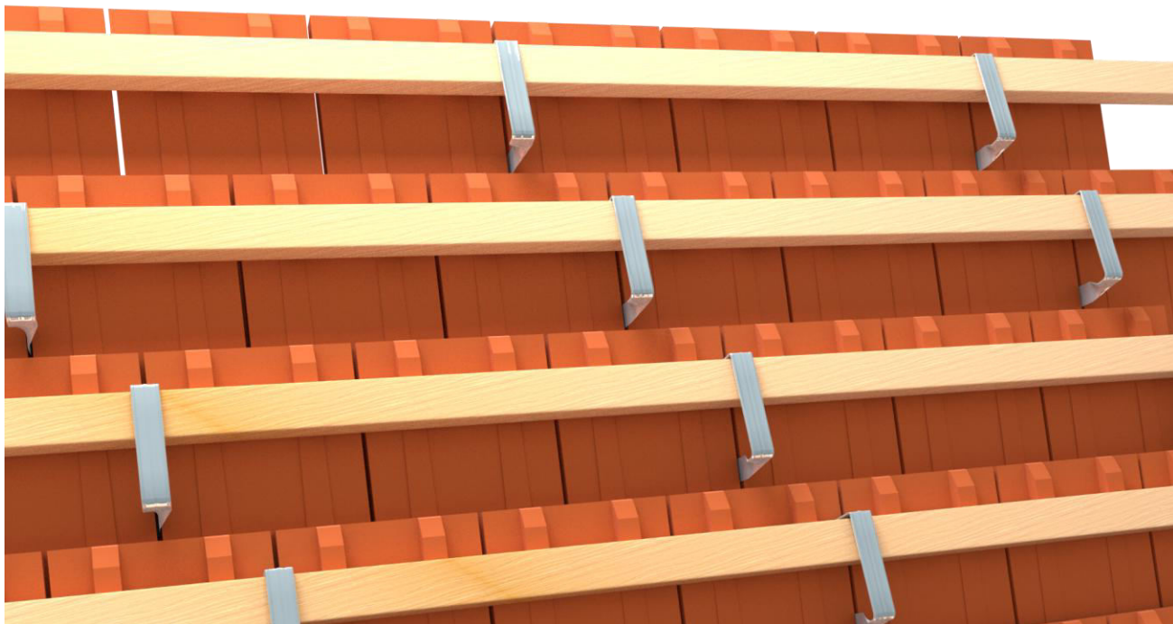
Séma 1:3 beakasztós viharokmányhoz, kettős-fedésű hódfarkú cserépfedéshez
