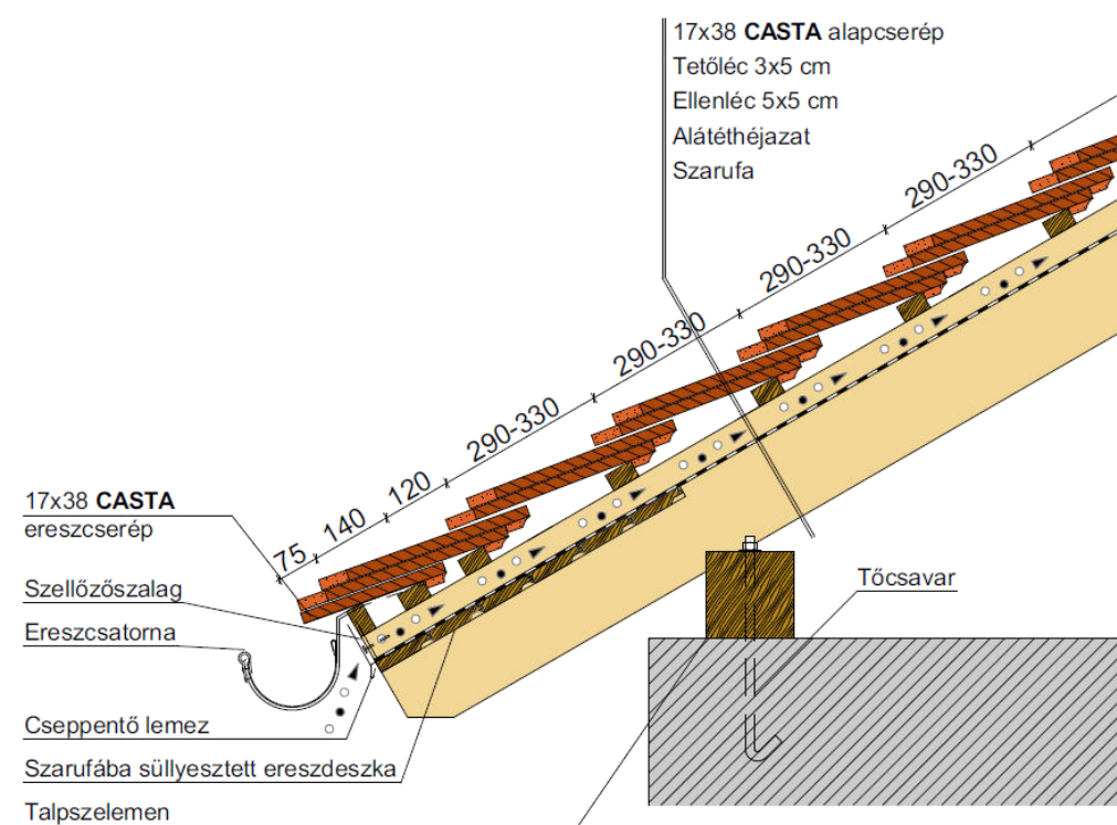
Koronafedésű ereszkialakítás
