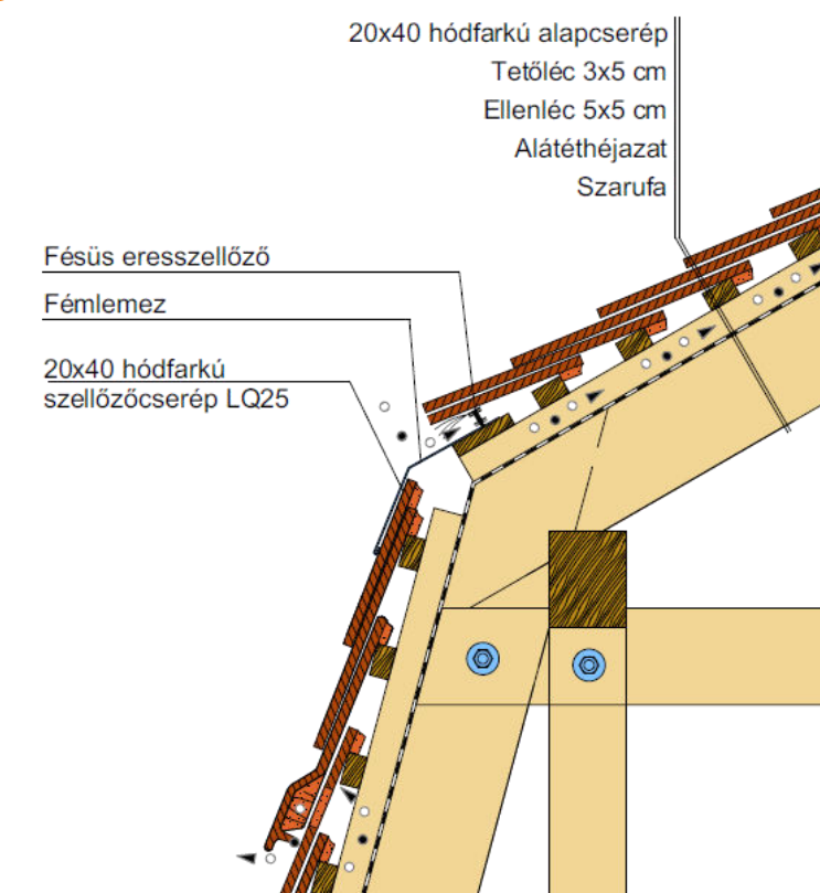
Negatív hajlásszögtörés kialakítás
