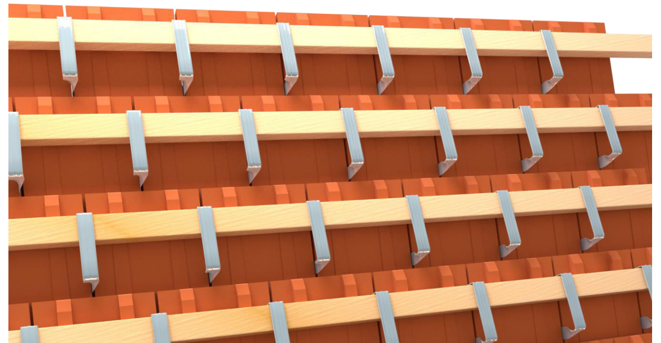
Séma 1:1 beakasztós viharokmányhoz, kettős-fedésű hódfarkú cserépfedéshez
