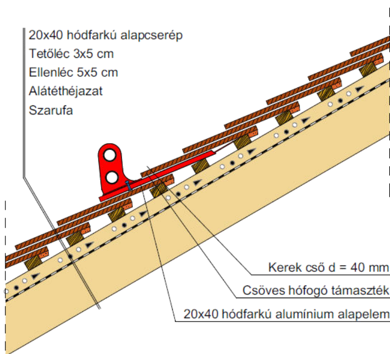
Rönkfartó elhelyezése
