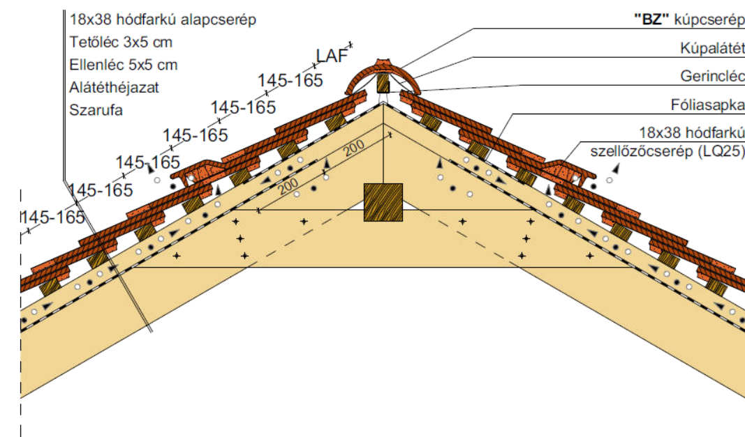
Gerinckialakítás, szellőzőcseréppel
