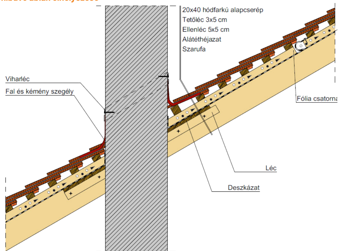
Kéményszegély kialakítás
