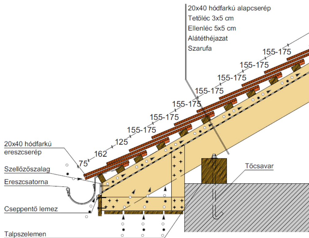
Dobozt ereszkialakítás
