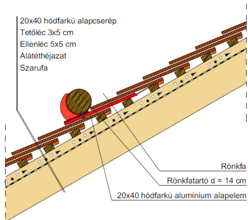
Rönkfartó elhelyezése
