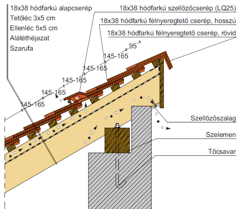
Félnyereggtető gerinc kialakítás, félnyereggtető cseréppel
