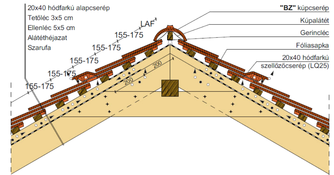
Gerinckialakítás, szellőzőcseréppel
