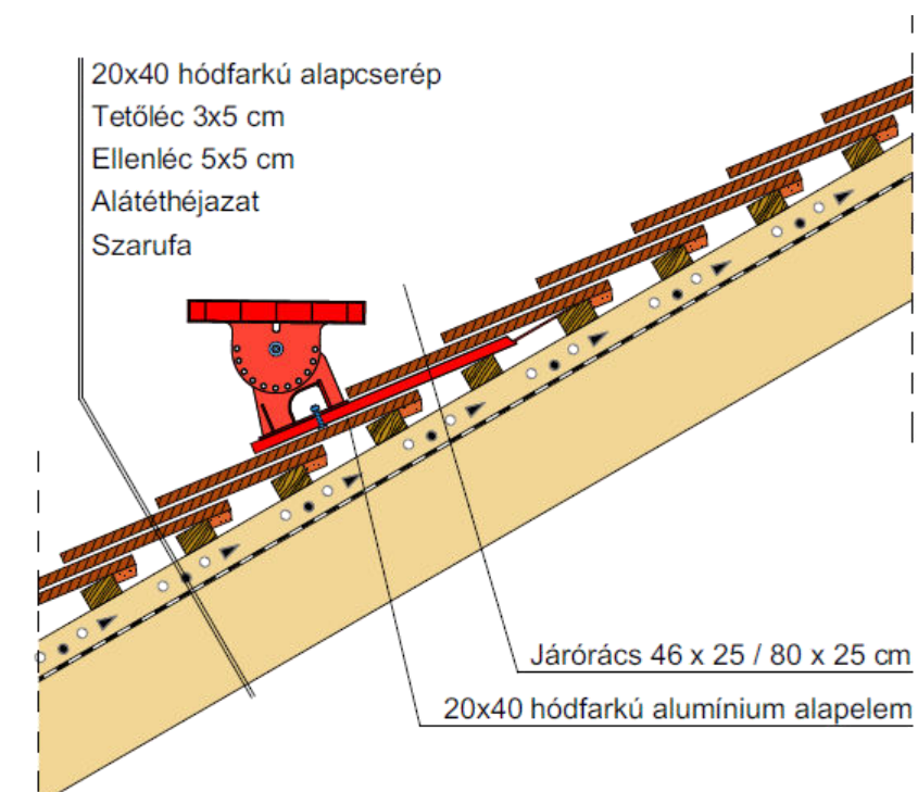
Járórács elhelyezése
