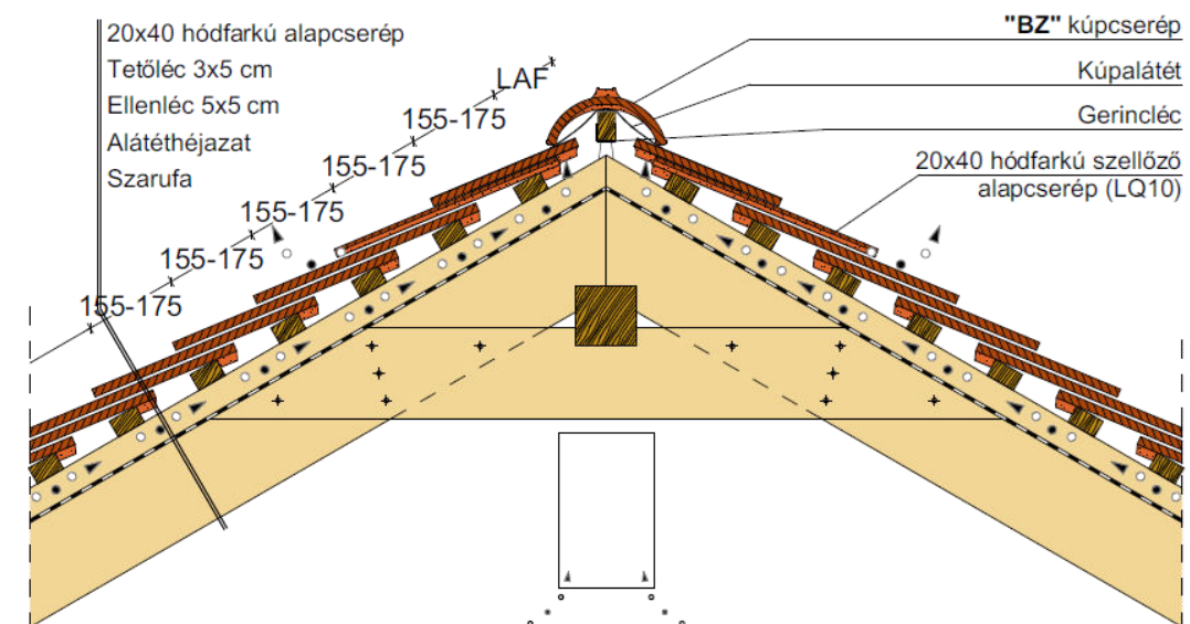
Gerinckialakítás, szellőző alapcsereppel
