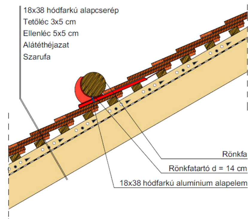
Rönkfartató elhelyezése
