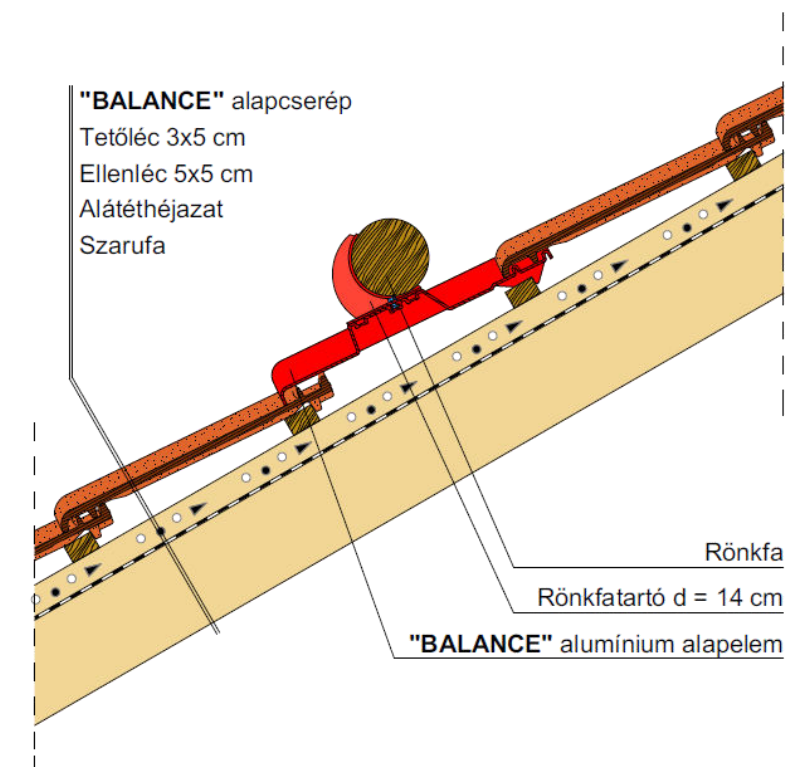
Rönkfartó elhelyezése
