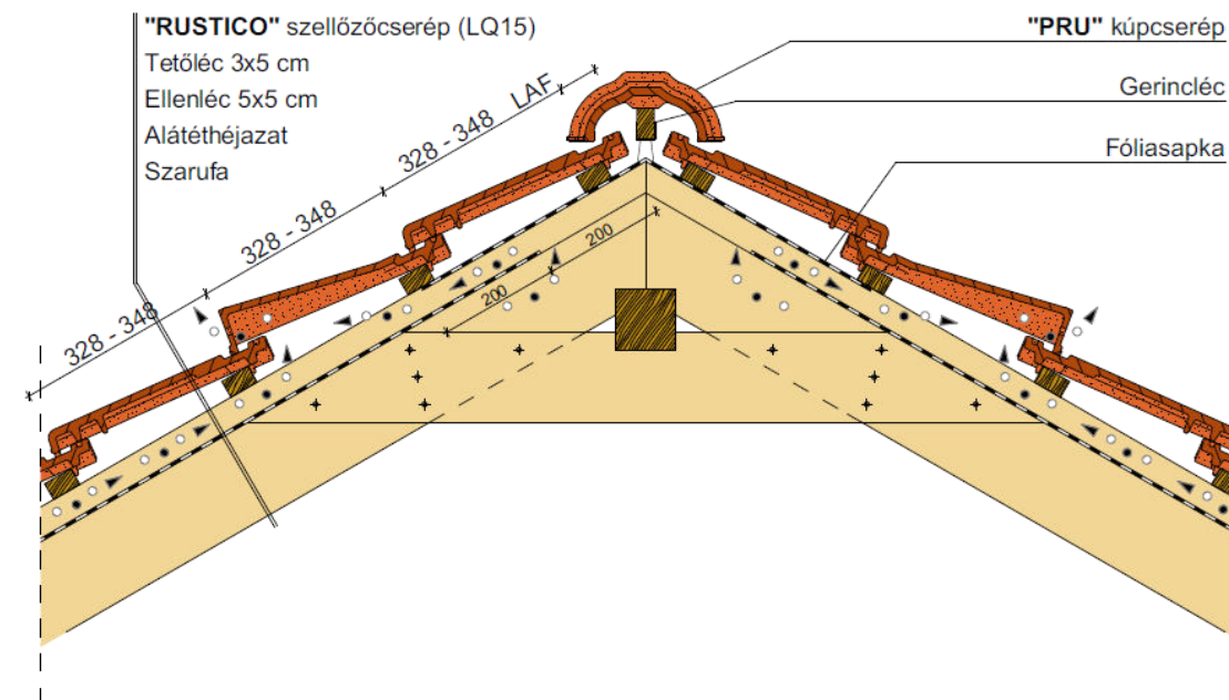
Gerinckialakítás, szellőzőcseréppel
