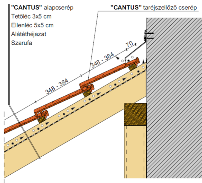
Falszegély kialakítás
