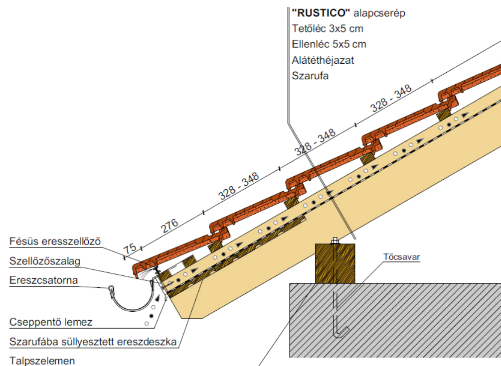
Ereszkialakítás
