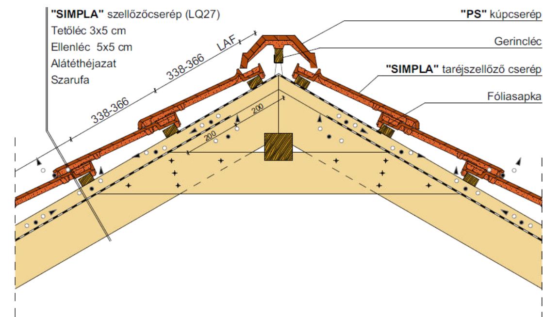
Gerinckialakítás, szellőzőcseréppel
