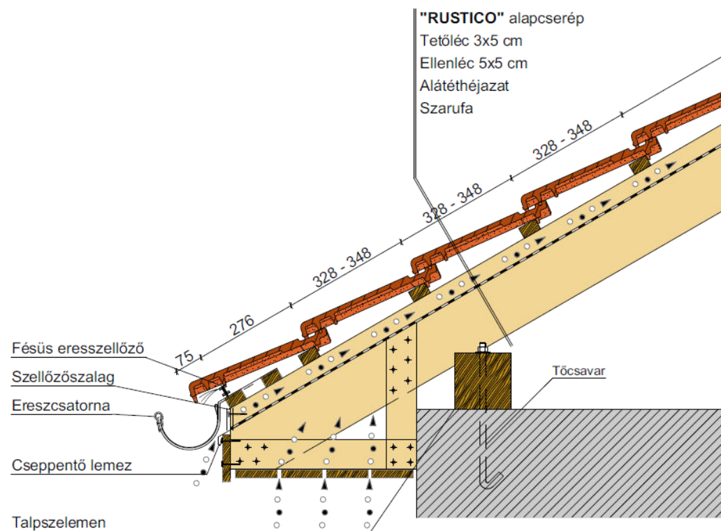
Dobozolt ereszkialakítás
