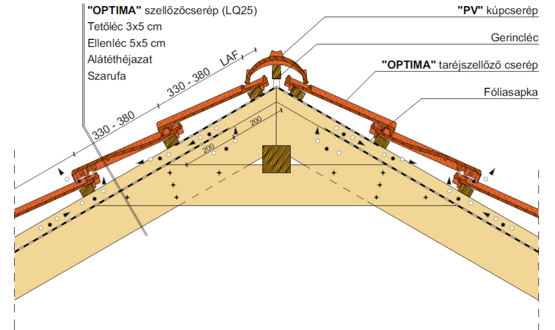
Gerinckialakítás, szellőzőcseréppel
