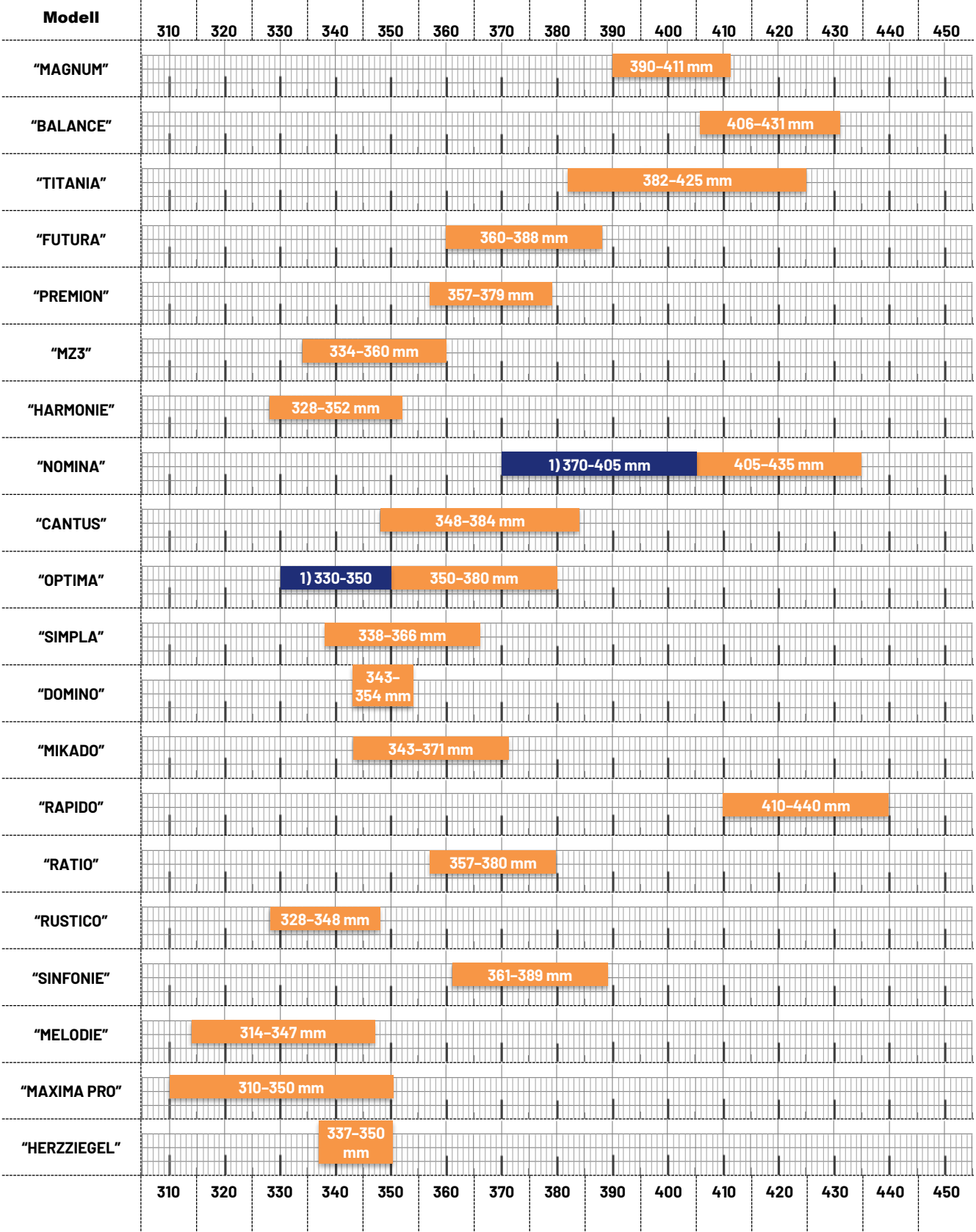
Léctávolságok [mm] áttekintése 1.) Az ábrázolt tartományban a szegélycserepek sarkát meg kell vágni!
