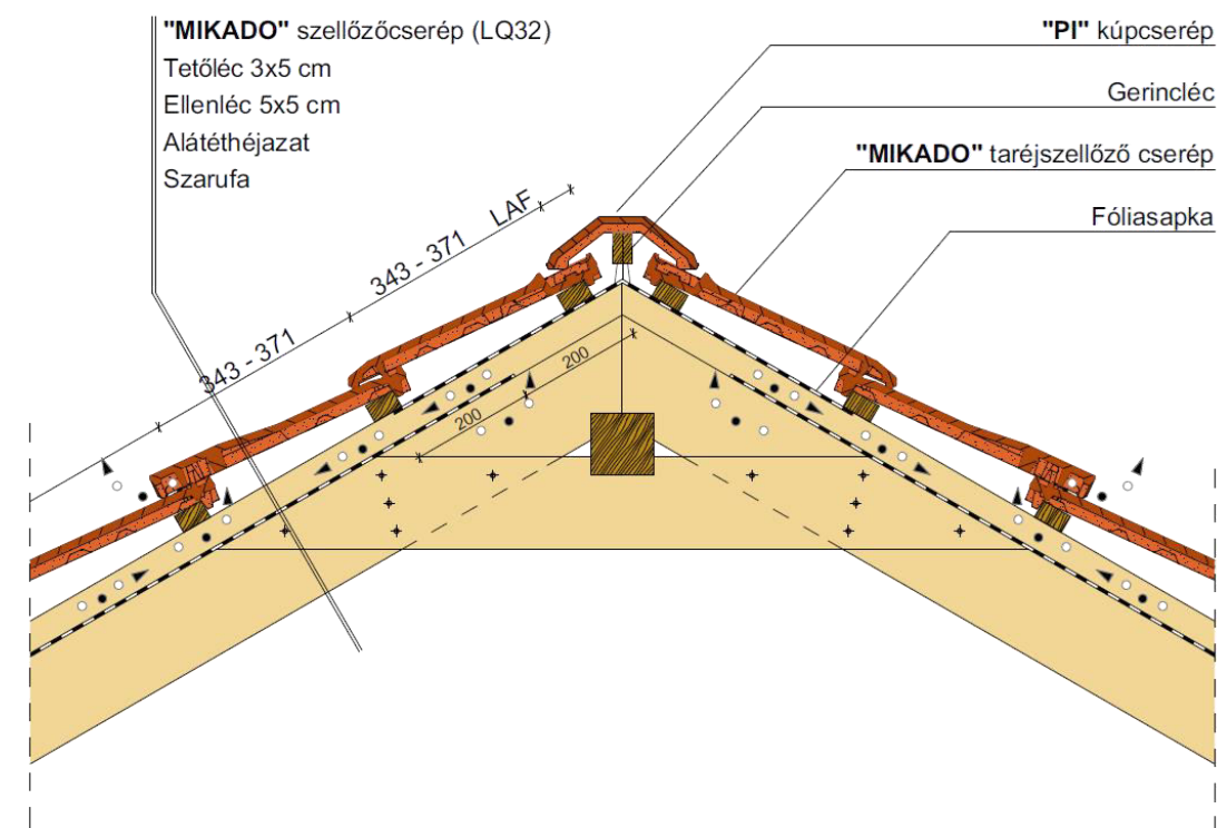
Gerinckialakítás, szellőzőcseréppel
