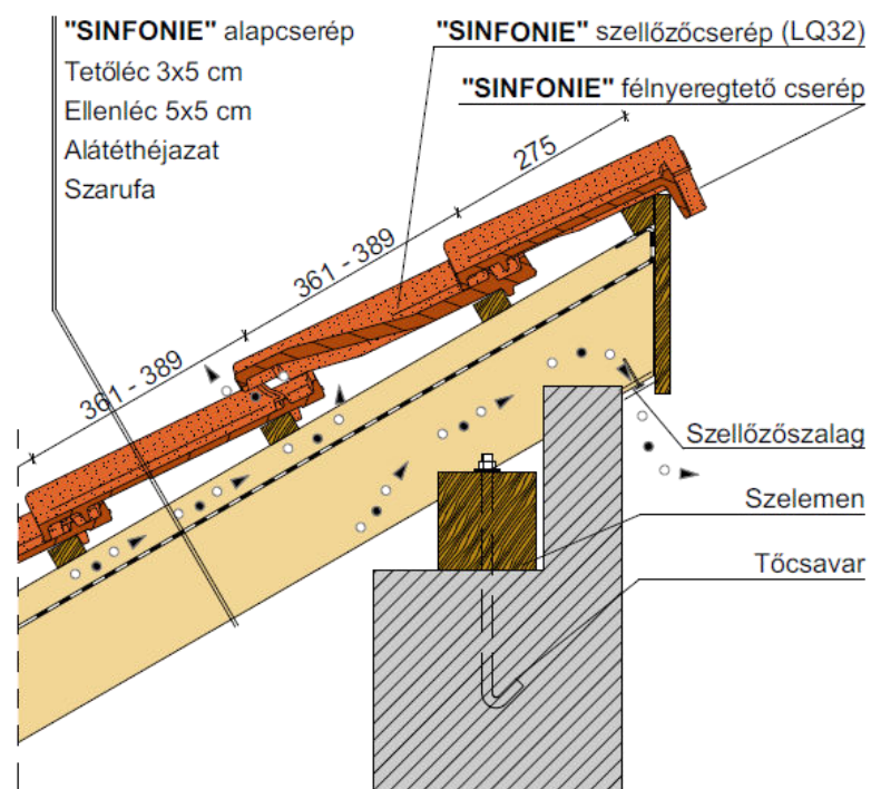
Félnyeregterítő gerinc, félnyeregterítő cseréppel
