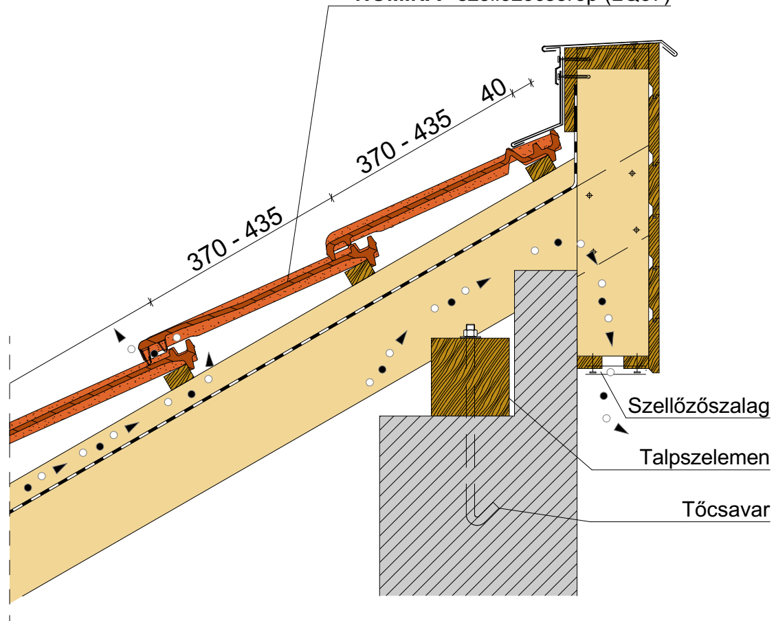
"NOMINA" szellőzőcserép (LQ37)
